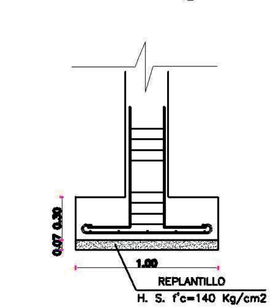
PLINTO TIPO 2
