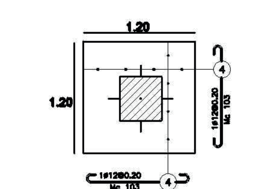
PLINTO TIPO 2
