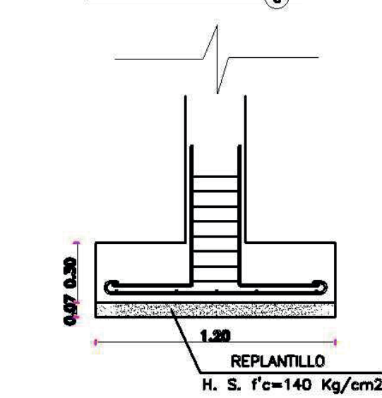
PLINTO TIPO 1
