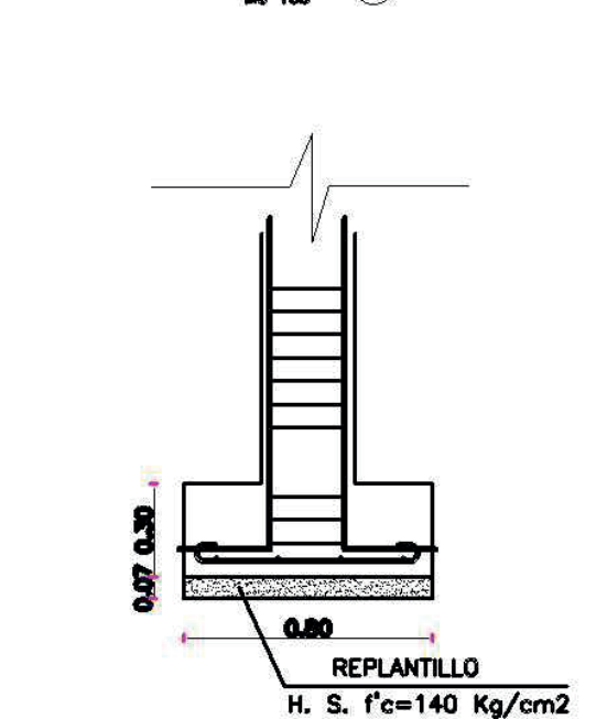
PLINTO TIPO 3
