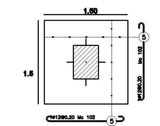
PLINTO TIPO 1
