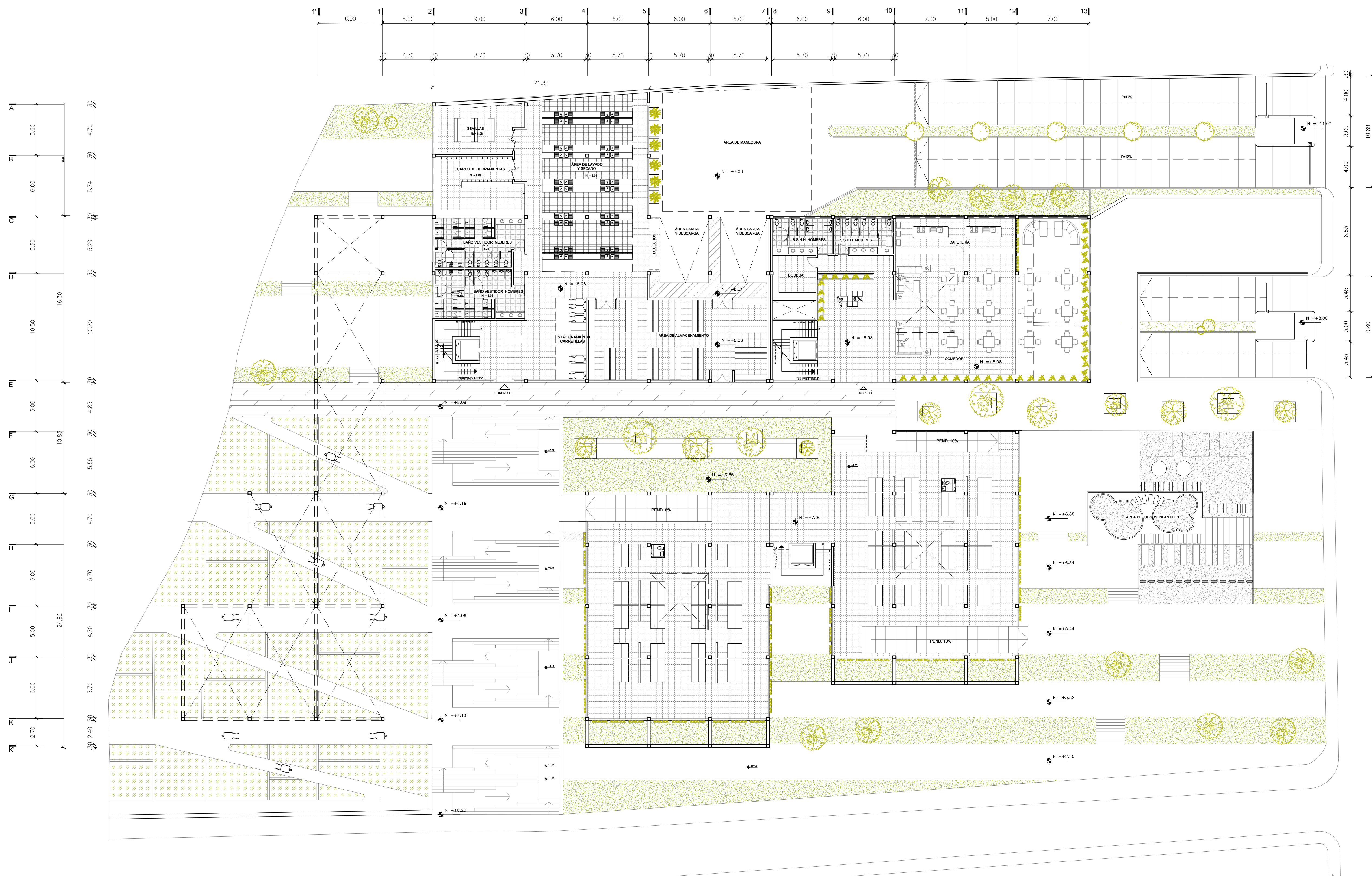
PLANTA ARQUITECTÓNICA N+7.06
