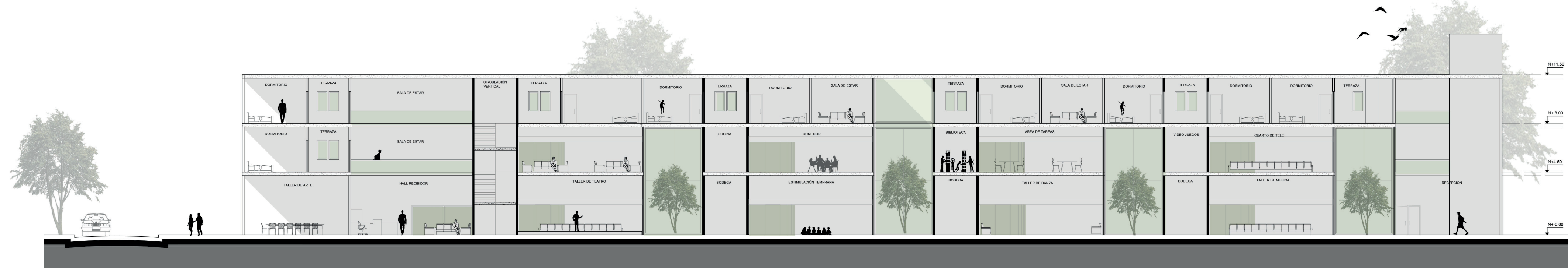
CORTE D - D' ESC 1---200
