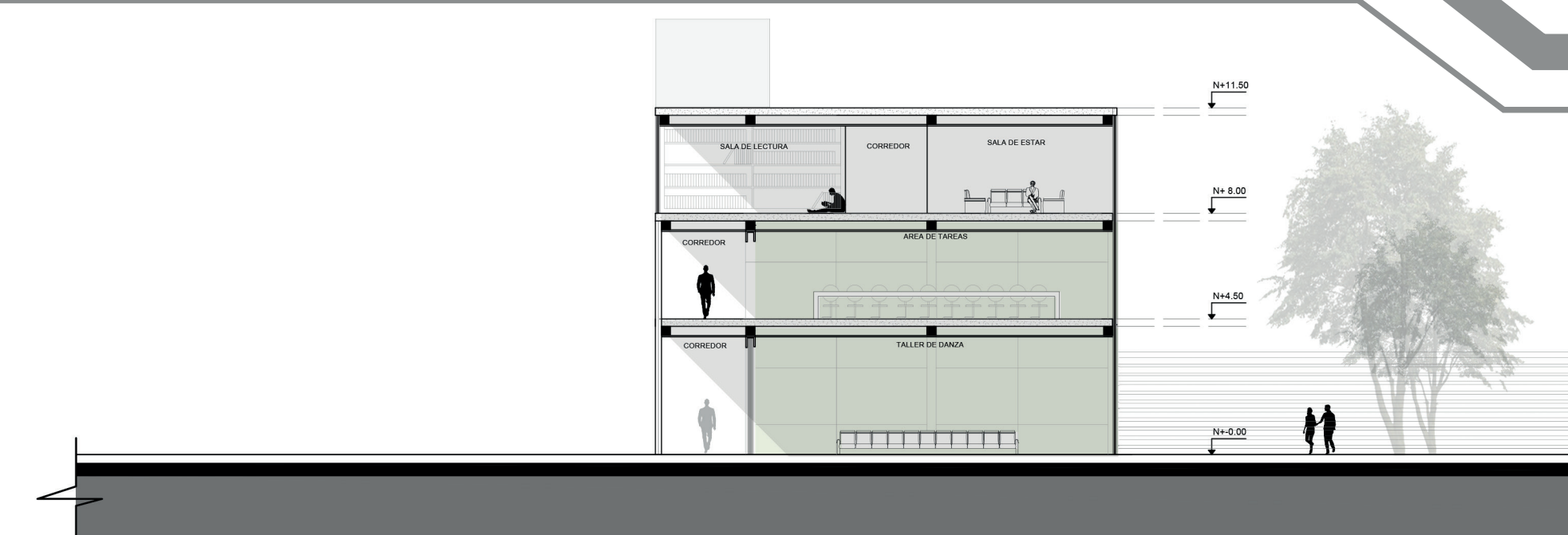
CORTE G - G' ESC 1---200
