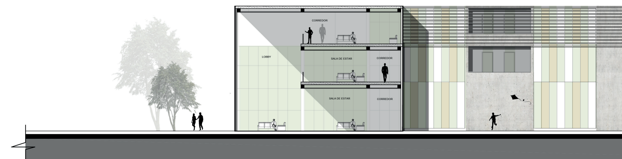
CORTE H - H' ESC 1---200
