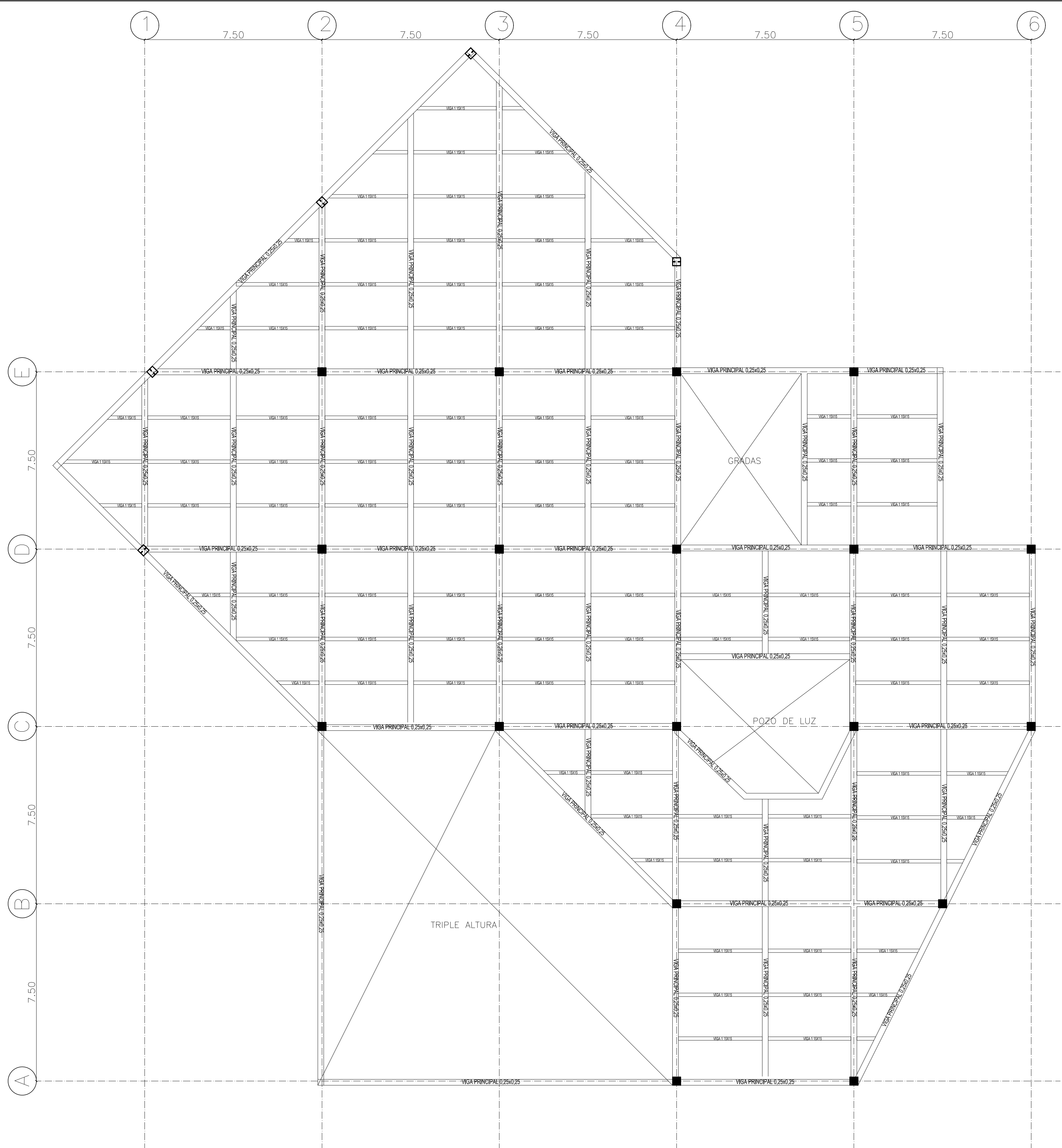
PLANTA DE VIGAS N + 4,50 ESCALA 1 : 100 CONSTRUCTIVA BLOQUE A
