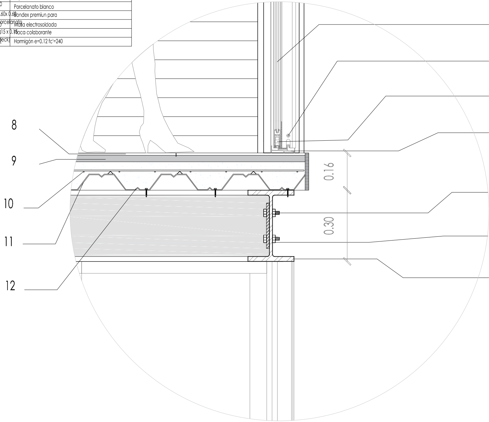
DETALLE 1 LOSA ESCALA 1 : 50 CONSTRUCTIVA BLOQUE A
