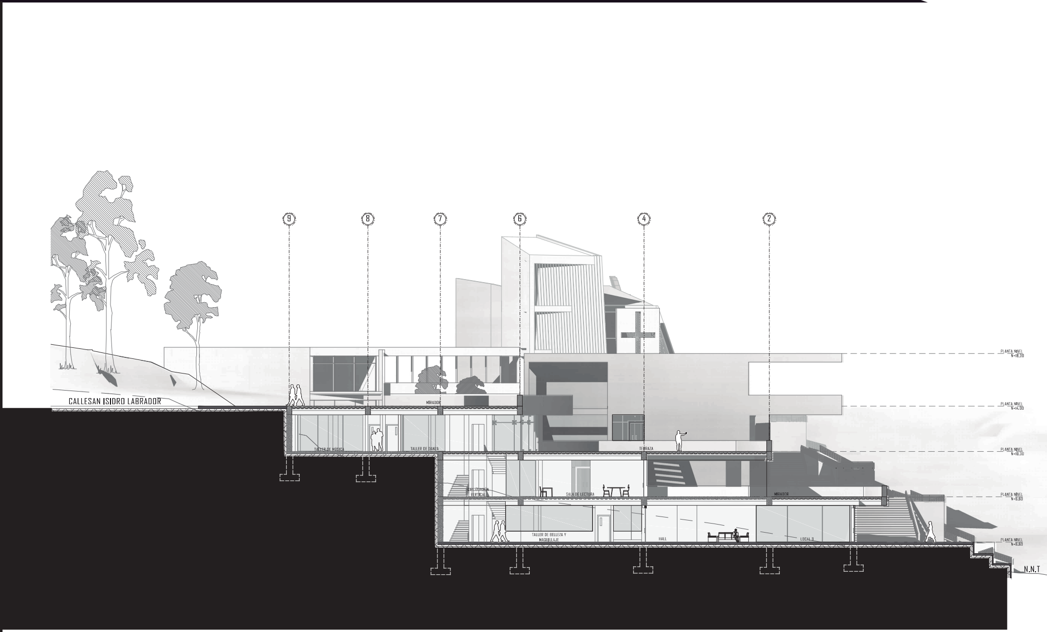
CORTE A-A' ESCALA GRÁFICA
