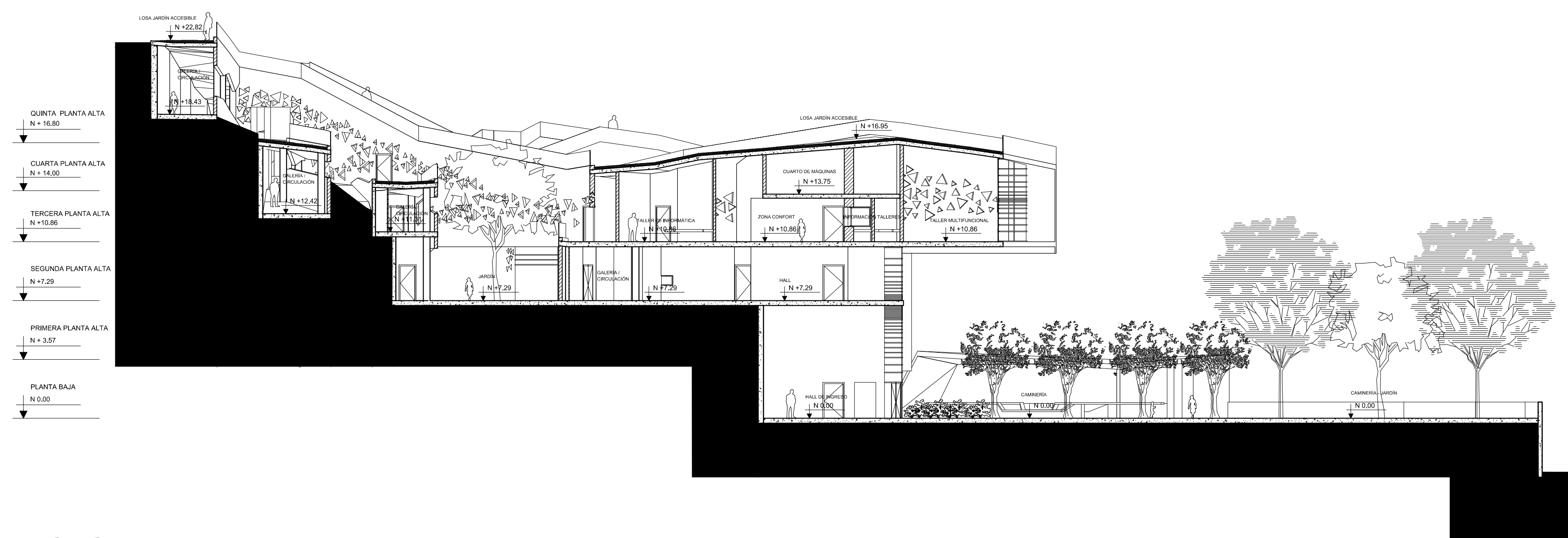
CORTE I-I'
