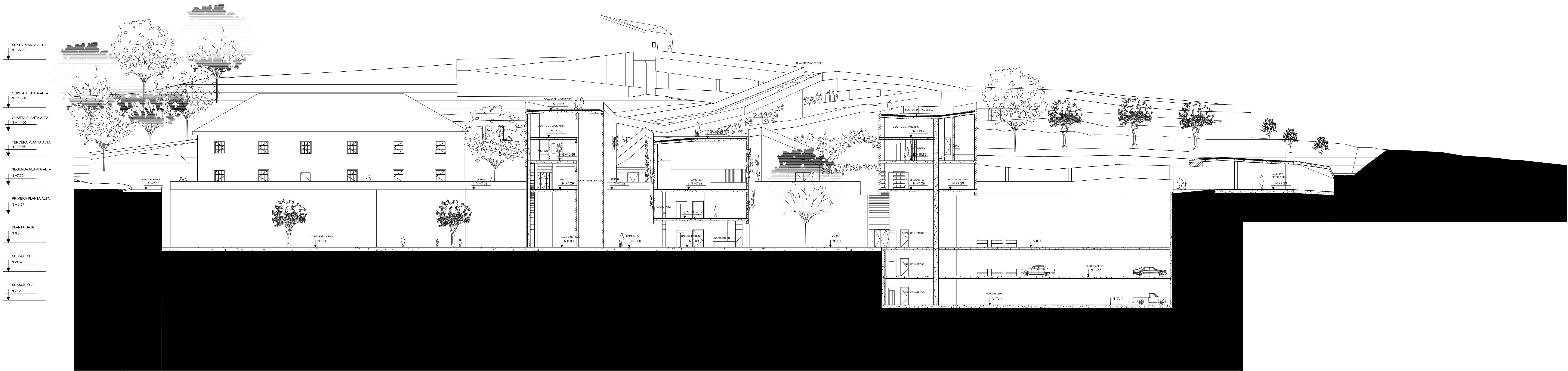
CORTE G-G'
