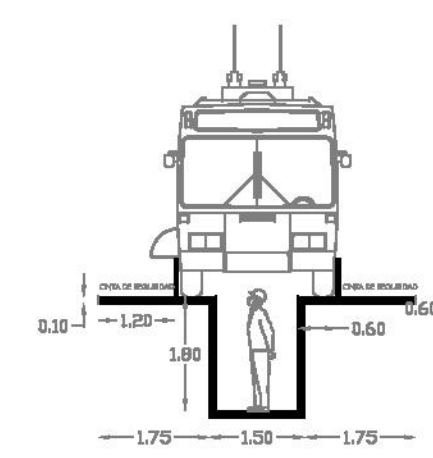
DETALLE FOSA TALLER MECANICO
