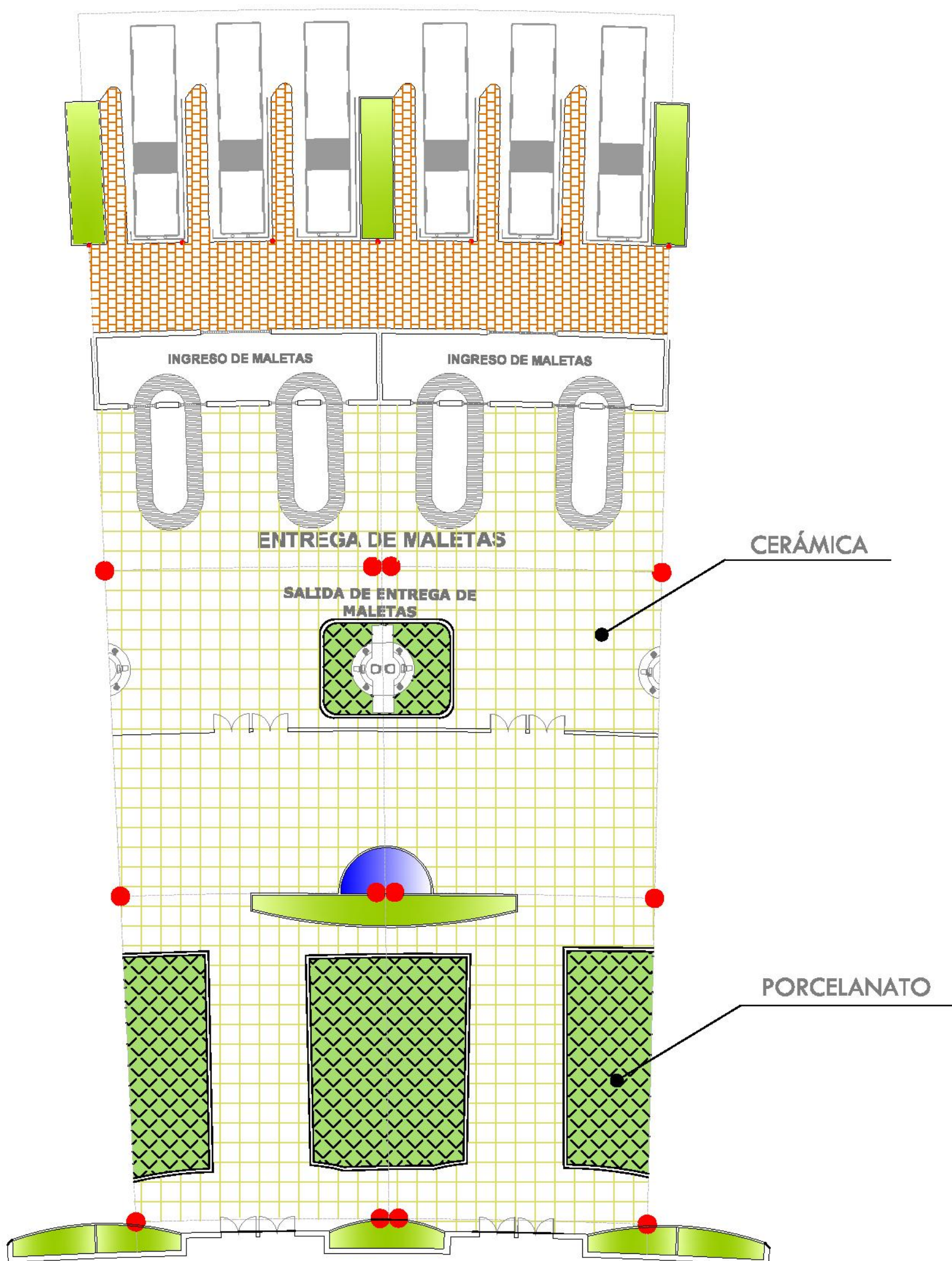
DETALLE PISO TERMINAL DE LLEGADA ESC. 1.25
