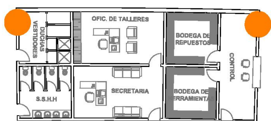
PLANTA AREA ADMINISTRATIVA DE TALLERES
