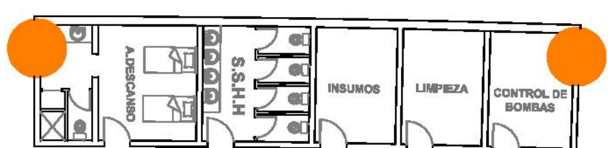
PLANTA AREA DE CONTROL Y DESCANSO GASOLINERA
