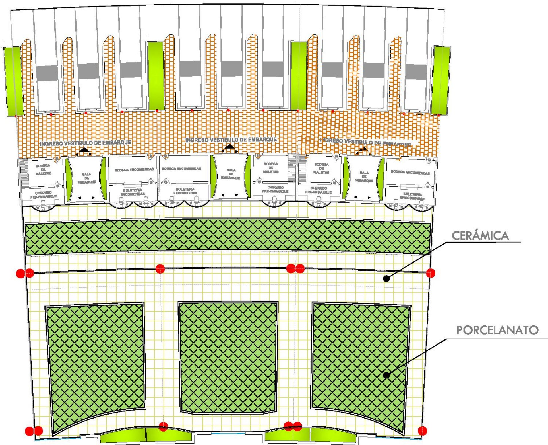
DETALLE PISO TERMINAL DE SALIDA ESC. 1.25
