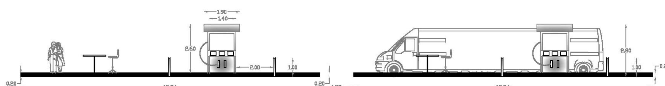
FACHADA DEL AREA DE DISTRIBUCION DE COMBUSTIBLE
