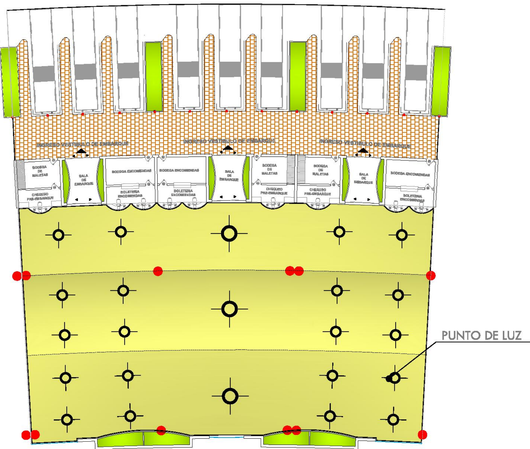
DETALLE TUMBADO TERMINAL DE SALIDA ESC. 1.25
