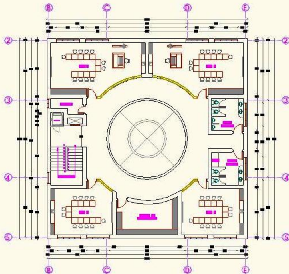
PLANTA ALTA DE CENTRO DE INTERPRETACIÓN ESC. 1:100
