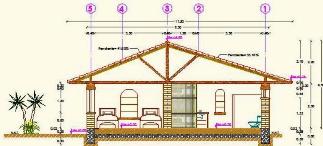
CORTE TRANSVERSAL VIVIENDA TIPO B (B-B)
