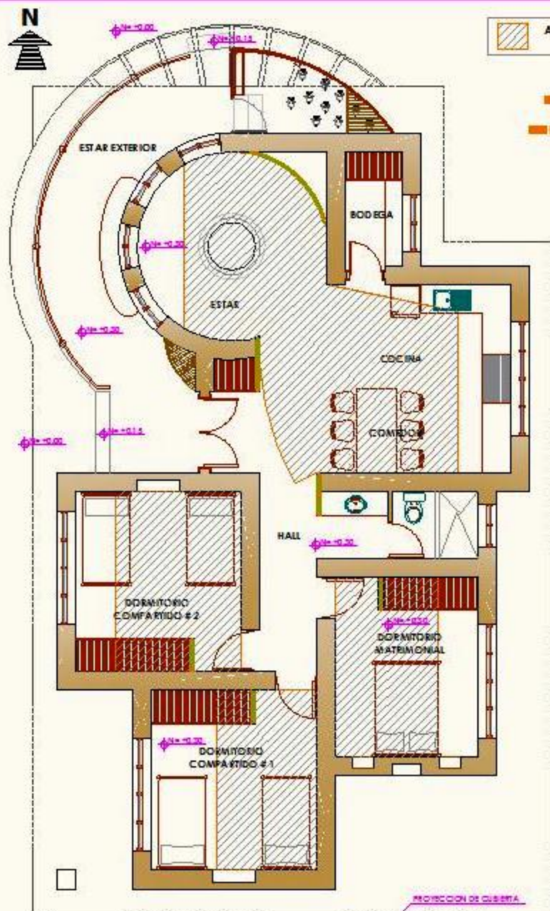
PLANTA VIVIENDA TIPO B ESC. 1:50
