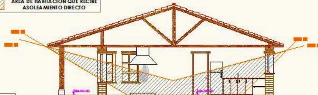
ESTAR, COCINA Y COMEDOR ESC. 1:50
