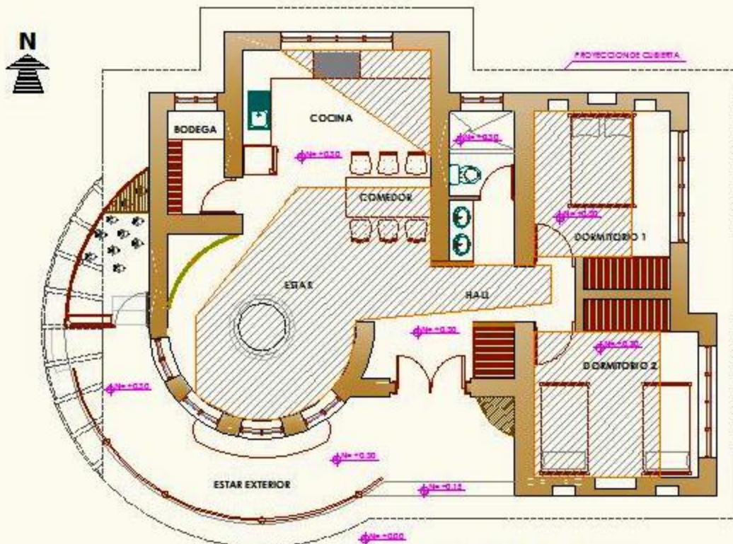
PLANTA VIVIENDA TIPO A
