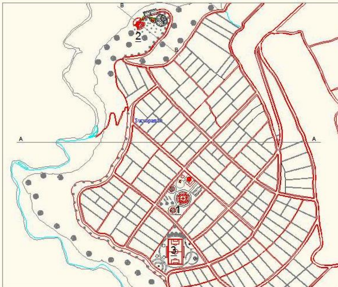
IMPLANTACIÓN GENERAL ESC. 1:2000
