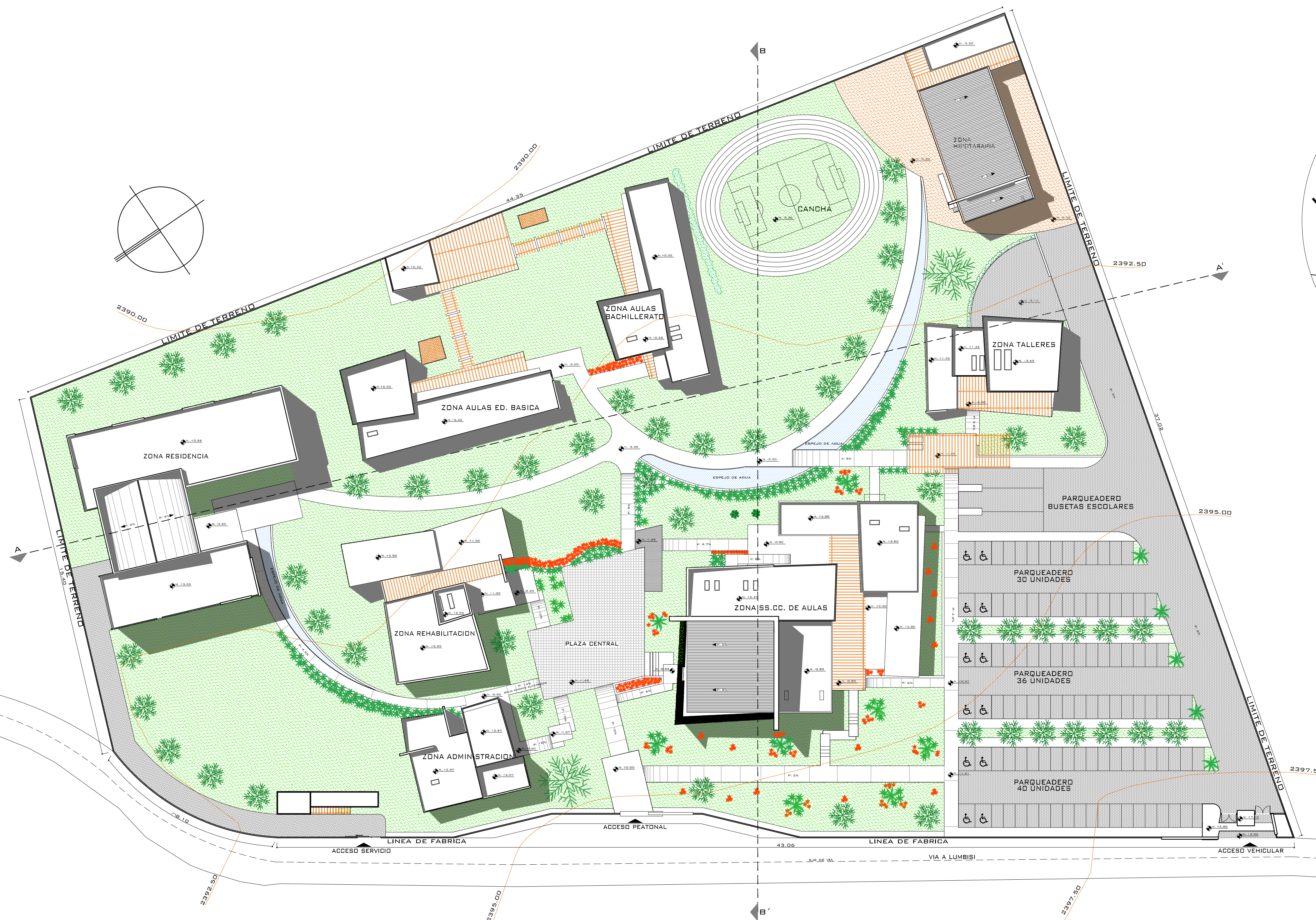
IMPLANTACION GENERAL DEL PROYECTO ESCALA:.....1:500
