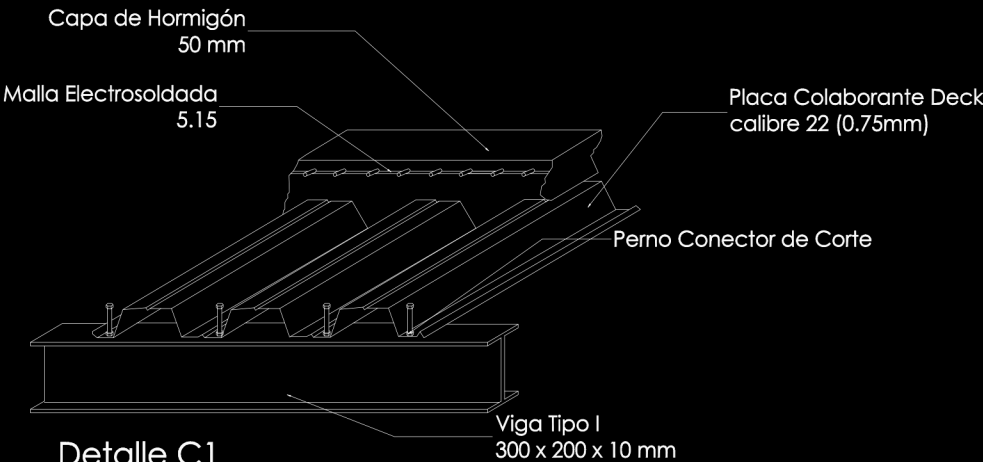
Detalle C1 Unión Placa Colaborante con Viga Tipo I Sin Escala
