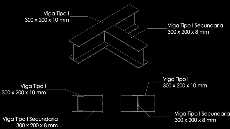
Detalle C3 Unión Viga Tipo I con Viga Tipo I Secundaria Sin Escala
