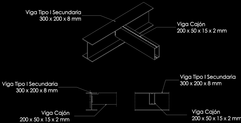
Detalle C4 Unión Viga Tipo I Secundaria con Viga Cajón Sin Escala
