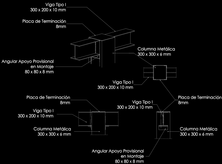
Detalle C2 Unión Columna Metálica con Viga Tipo I Sin Escala
