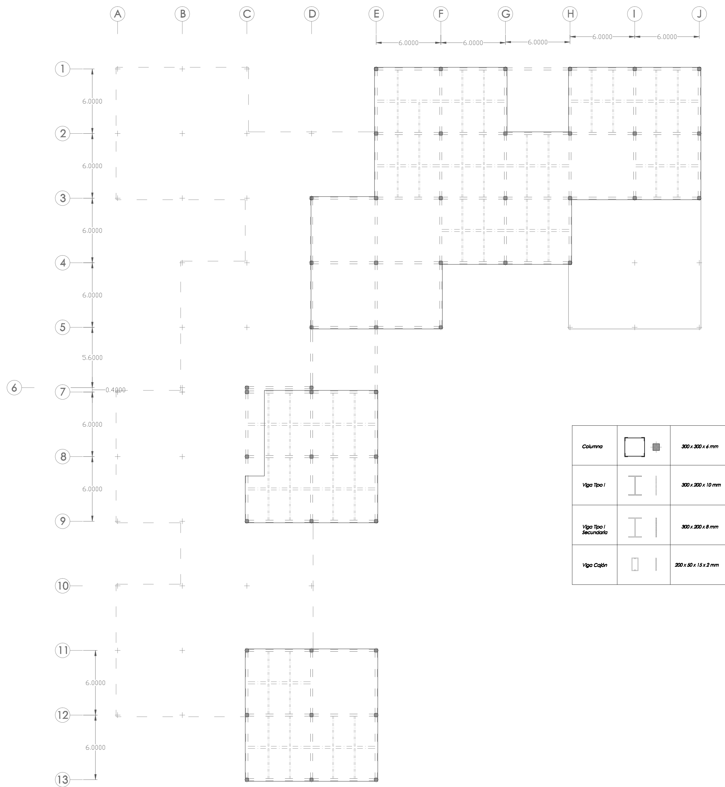
PLANTA PRIMERA Nivel +9.40 Esc. 1:200
