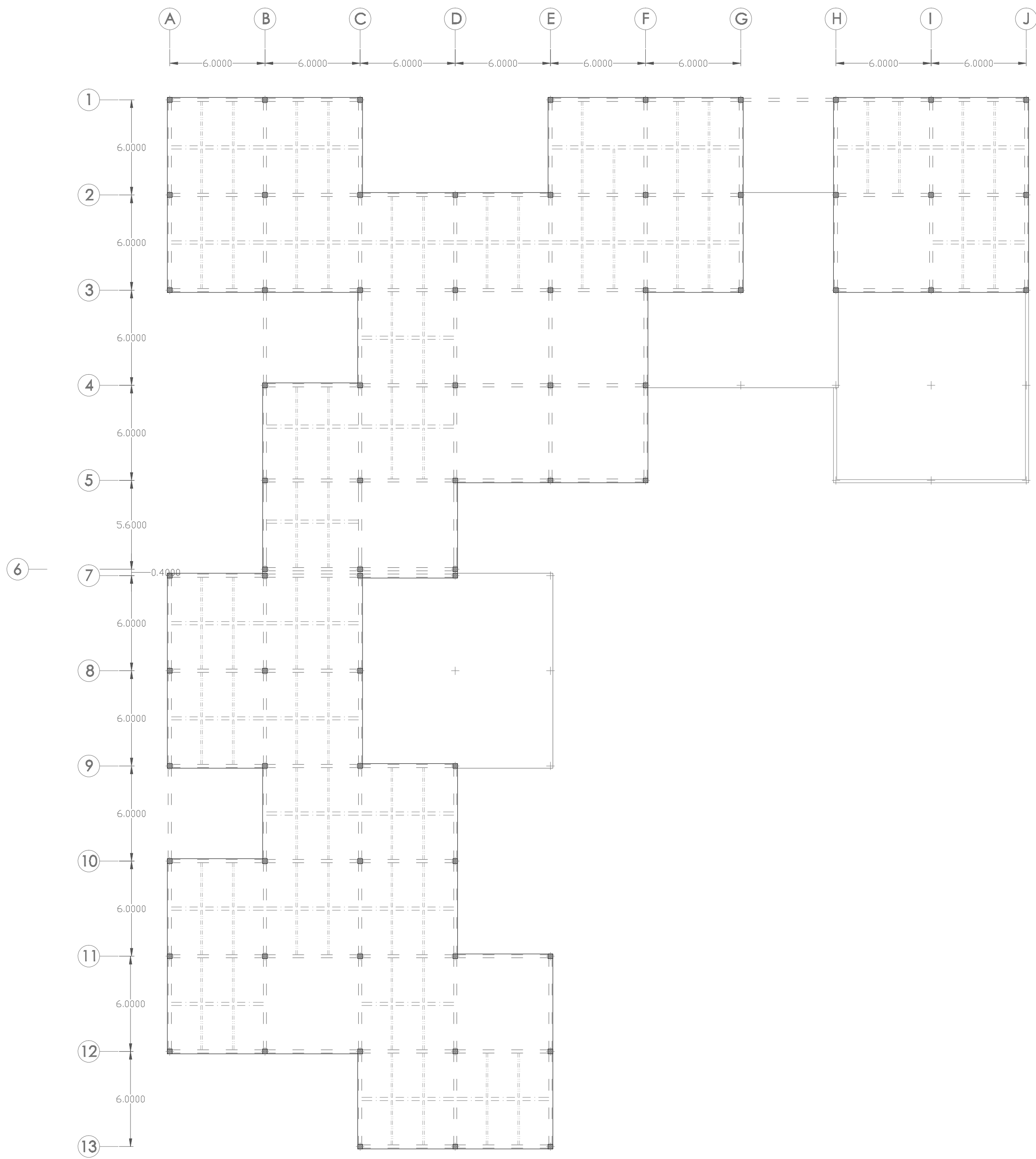
PLANTA SEGUNDA Nivel +12.80 Esc. 1:200
