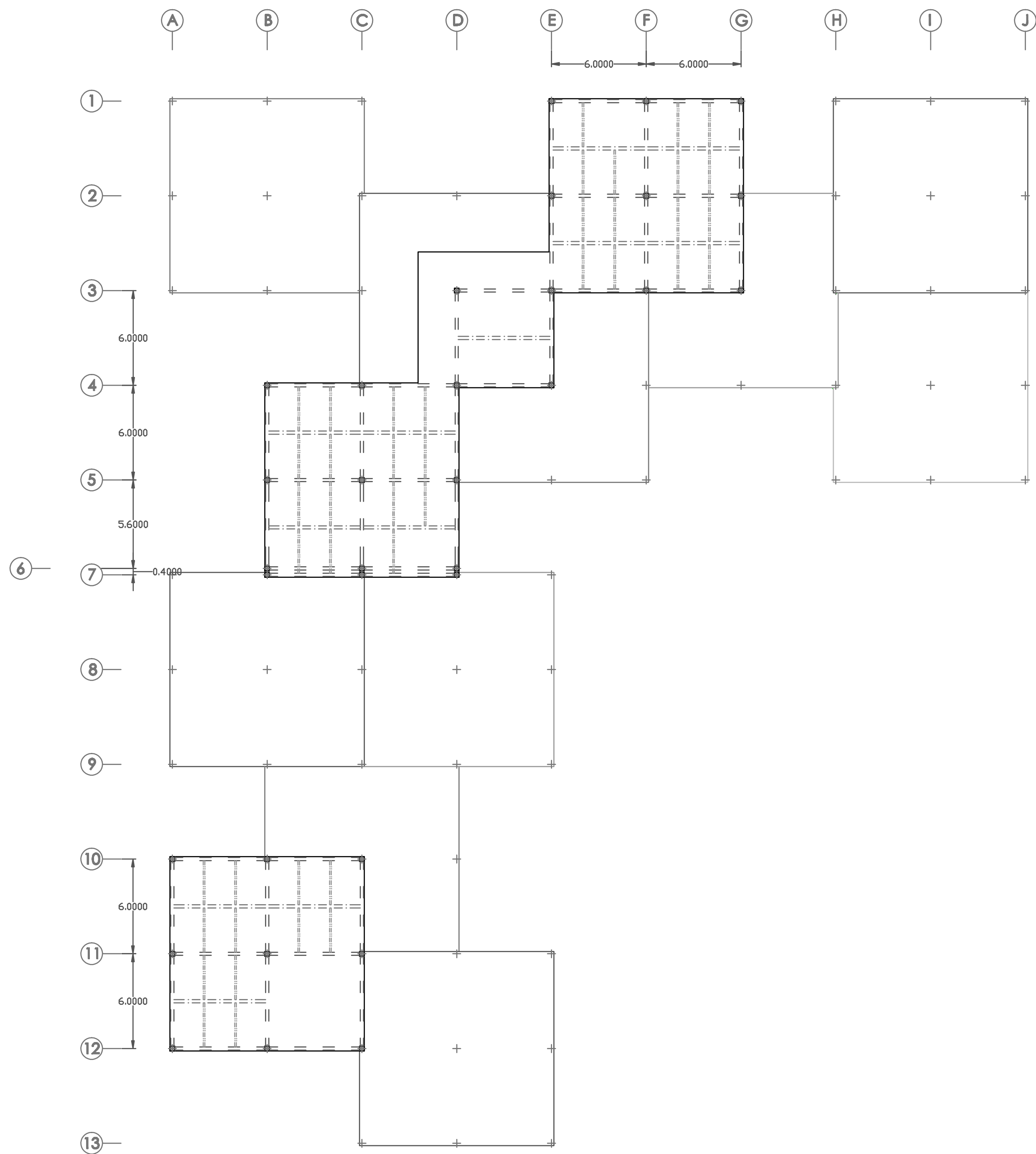
PLANTA CUARTA Nivel 19.60 Esc. 1:200
