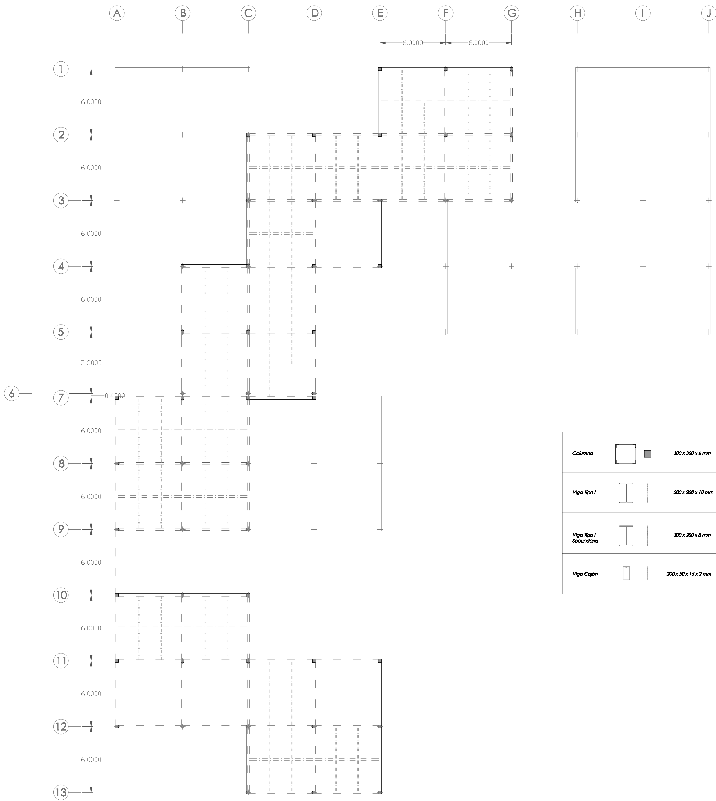
PLANTA TERCERA Nivel 16.20 Esc. 1:200
