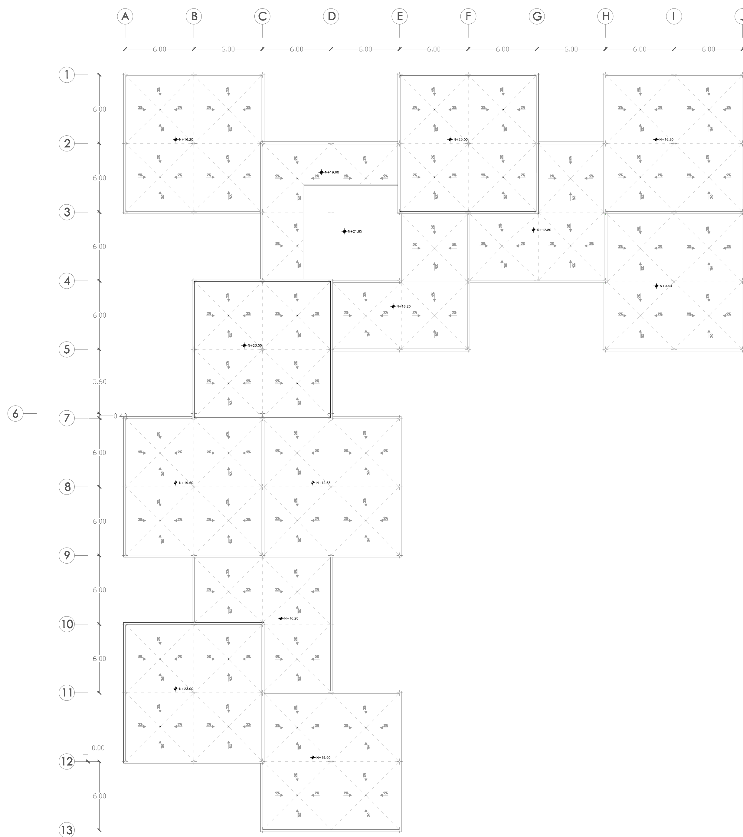
PLANTA CUBIERTAS Nivel 23.00 Esc. 1:200
