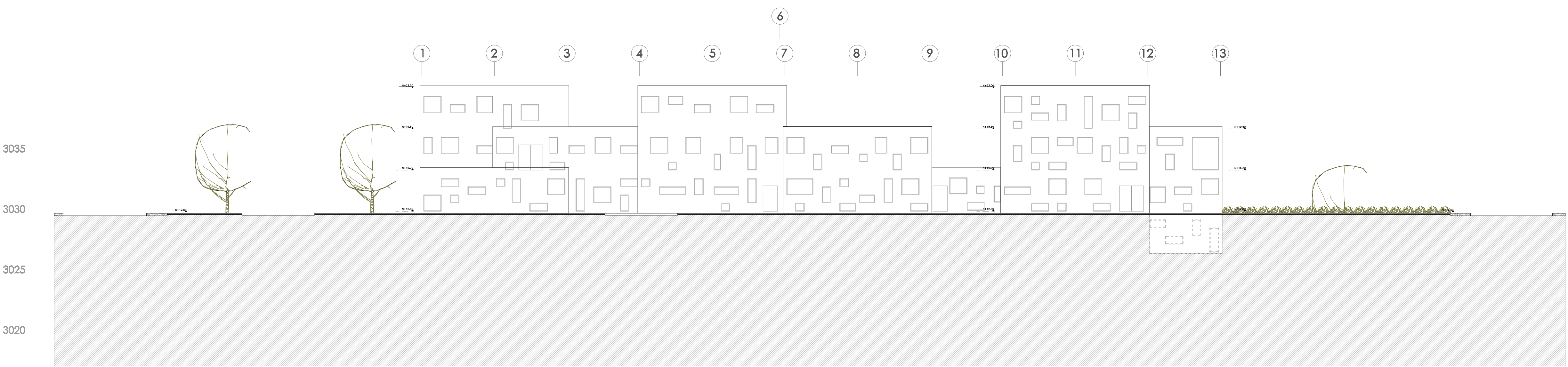
CORTE K - K' Fachada Oeste Esc. 1:200
