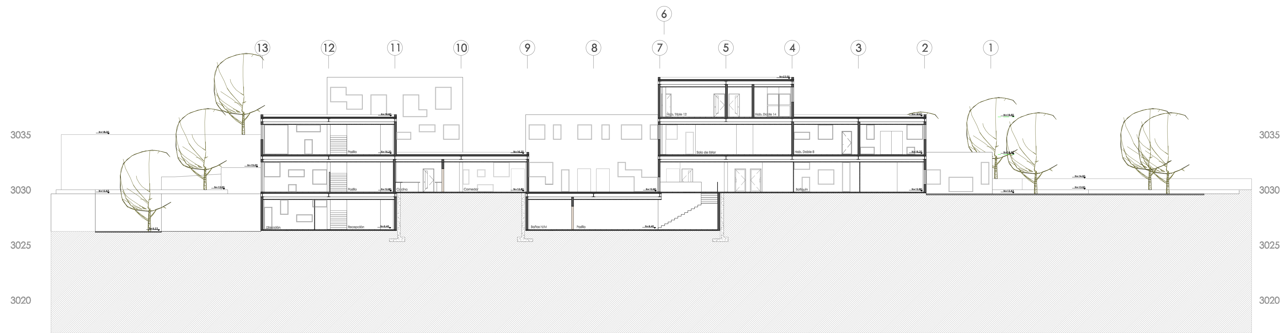
CORTE I - I' Esc. 1:200
