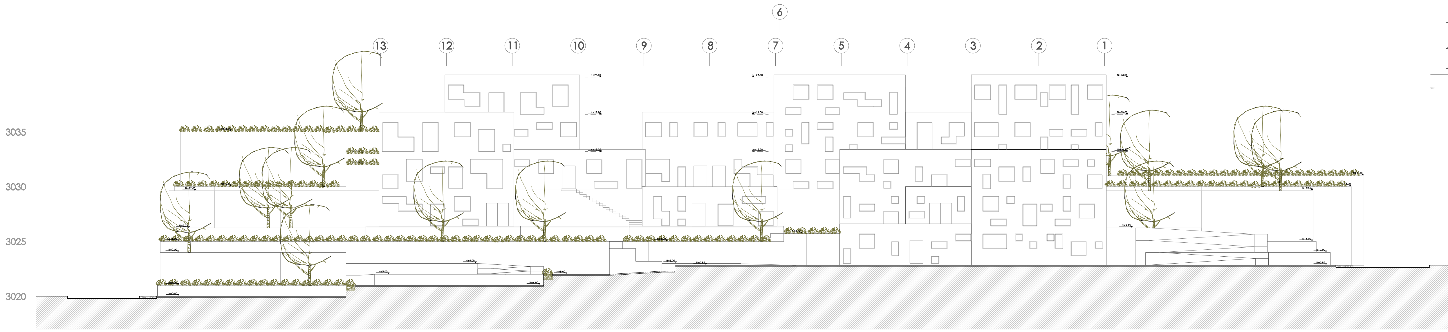
CORTE J - J' Fachada Este Esc. 1:200
