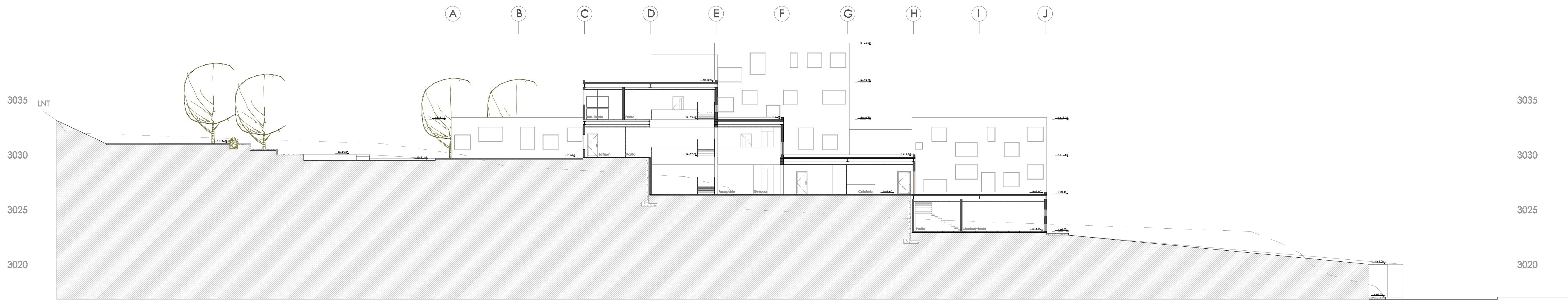
CORTE F - F' Esc. 1:200
