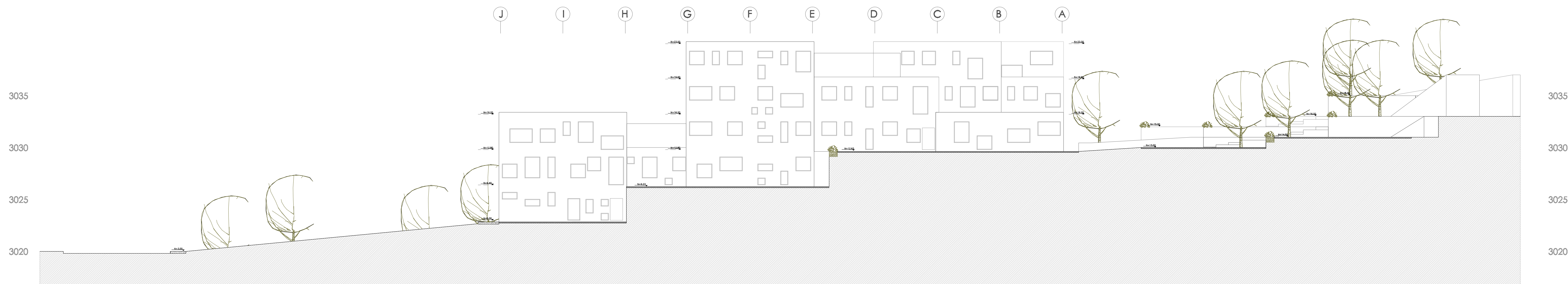
CORTE H - H' Fachada Norte Esc. 1:200
