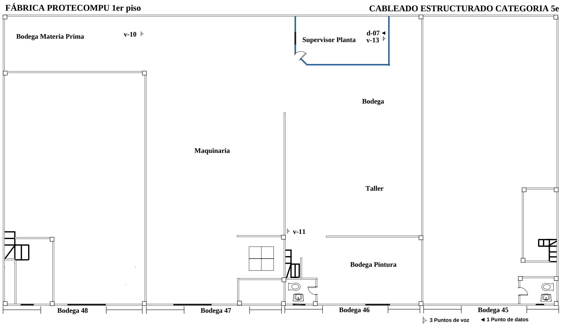
Figura. 2.12 Planos de la ubicación de los puntos de voz y datos primer piso
