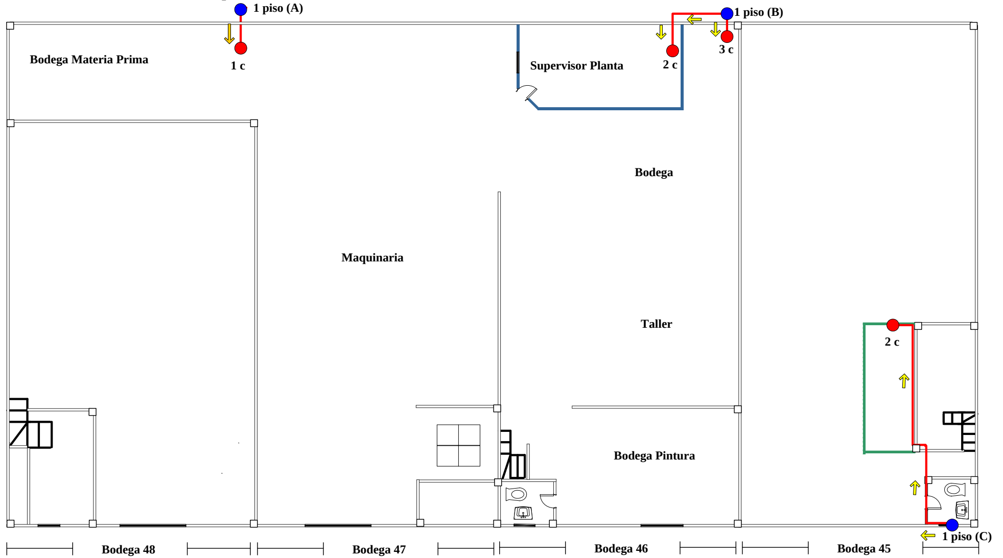
Figura. 3.3 Diseño de rutas de tubería y cable UTP del Sistema de Cableado Estructurado Primer Piso
