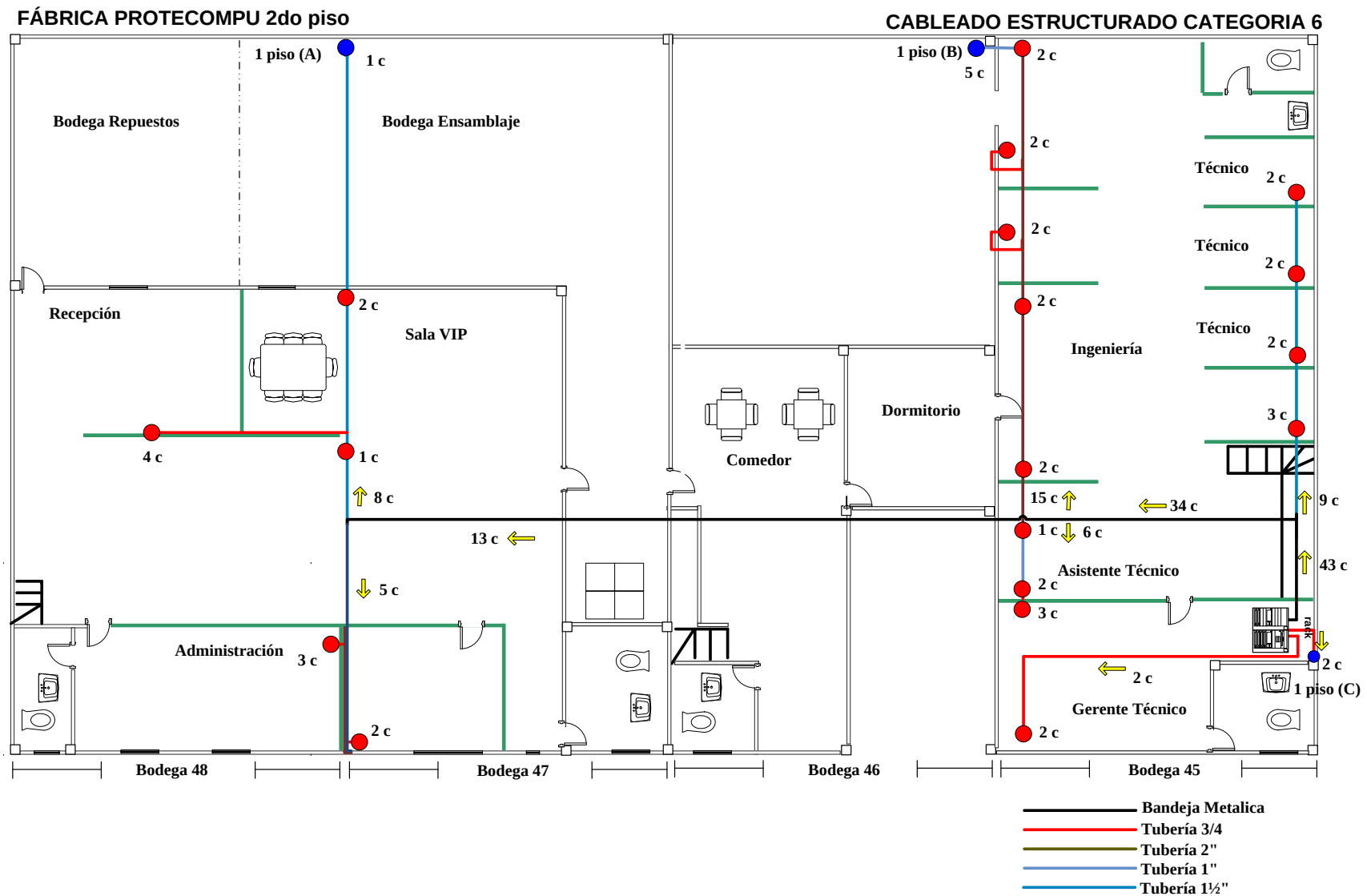
Figura. 3.4 Diseño de rutas de tubería y cable UTP del Sistema de Cableado Estructurado Segundo Piso
