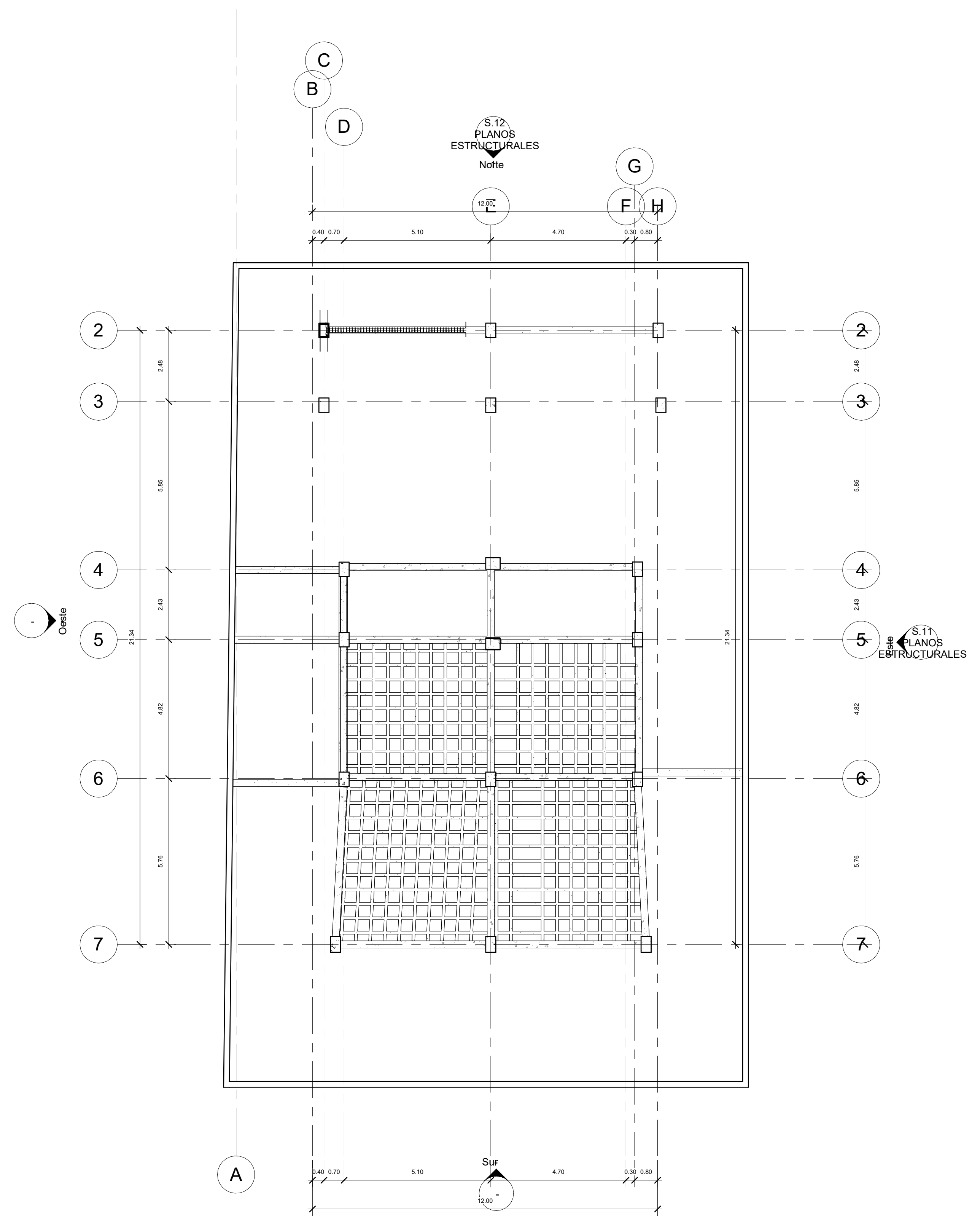
1 N-1.68 RAMPA 1 : 100
