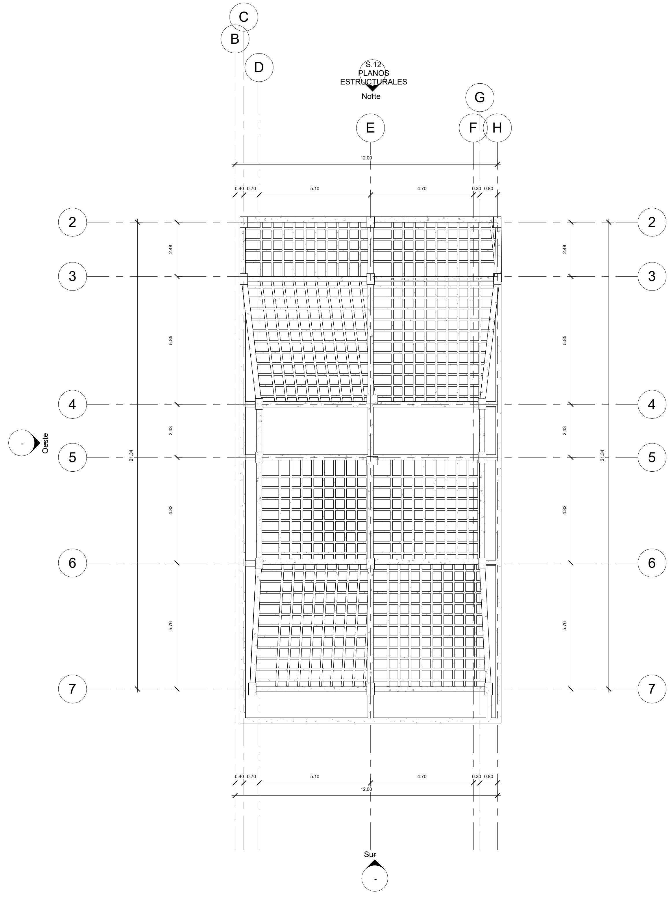
1 Nivel 5 1 : 100
