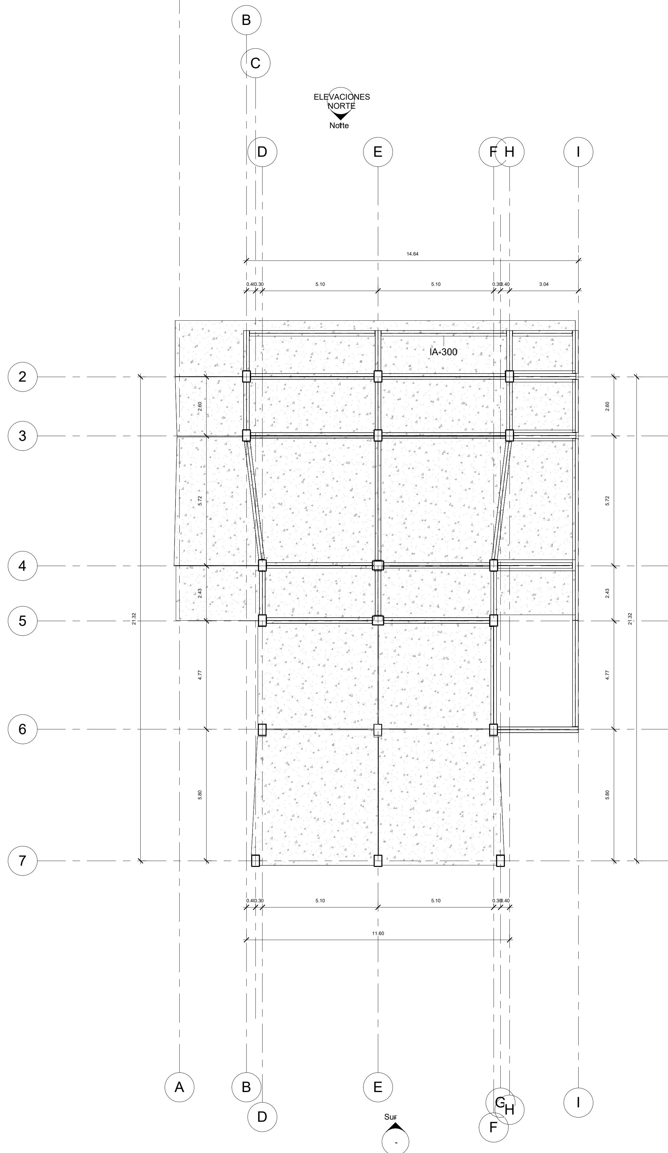
1 N-1.68 RAMPA PB 1 : 100
