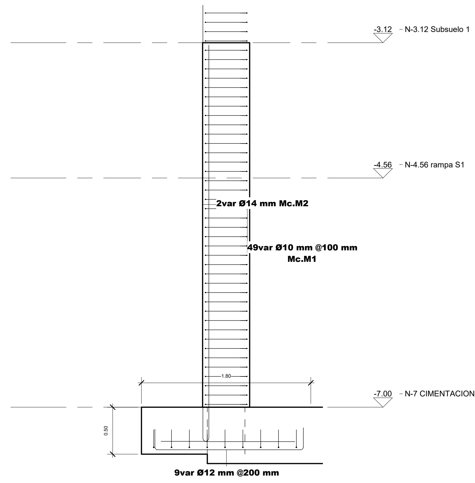
6 DETALLE DE ACERO EN COLUMNA 1 : 25
