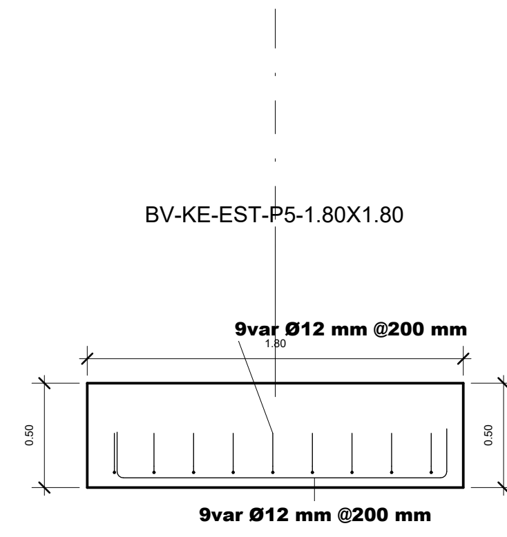
7 Sección 1 CIMENTACION 1 : 25
