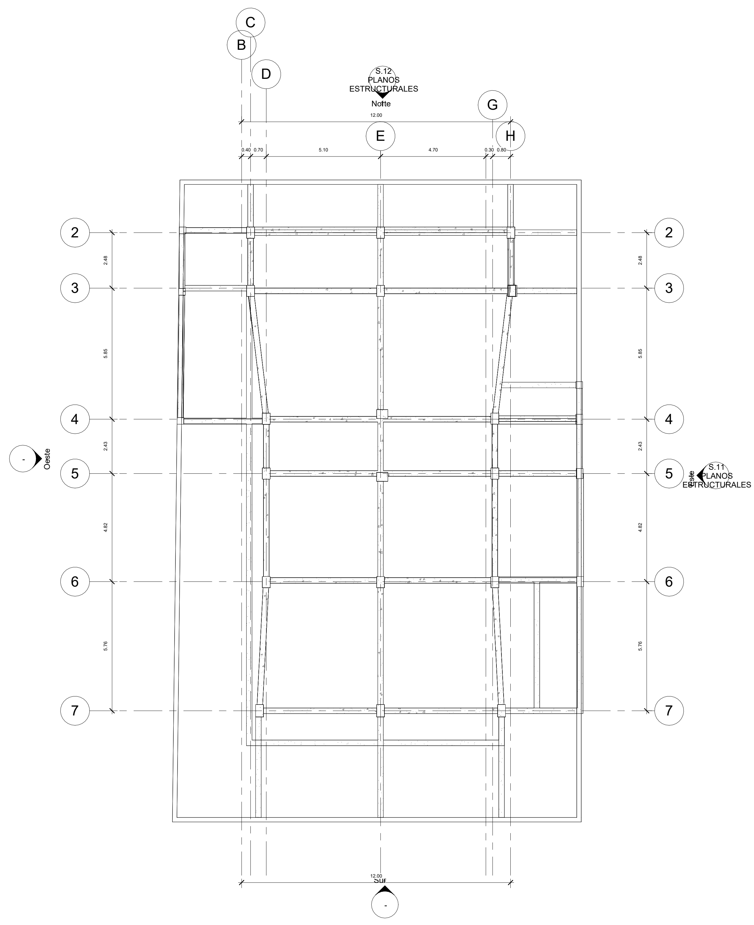
1 Nivel 2 1 : 100
