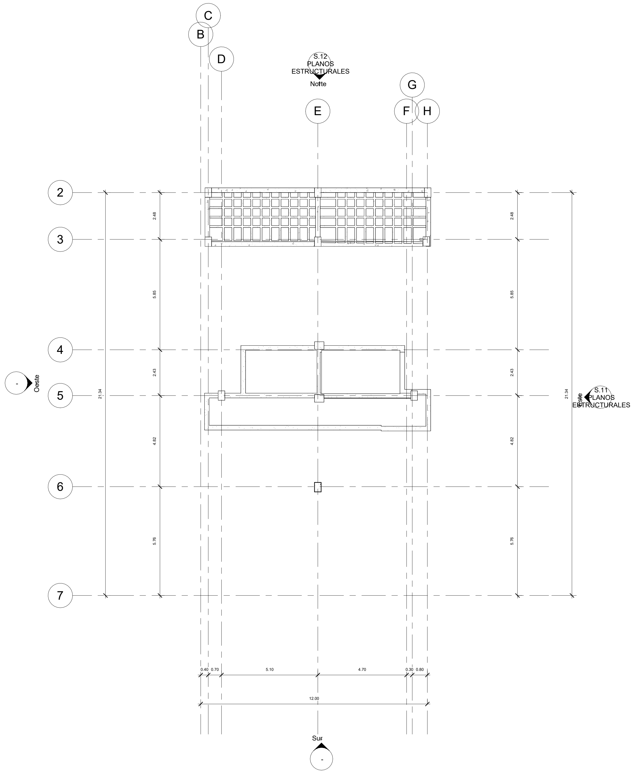
1 Nivel 6 1 : 100
