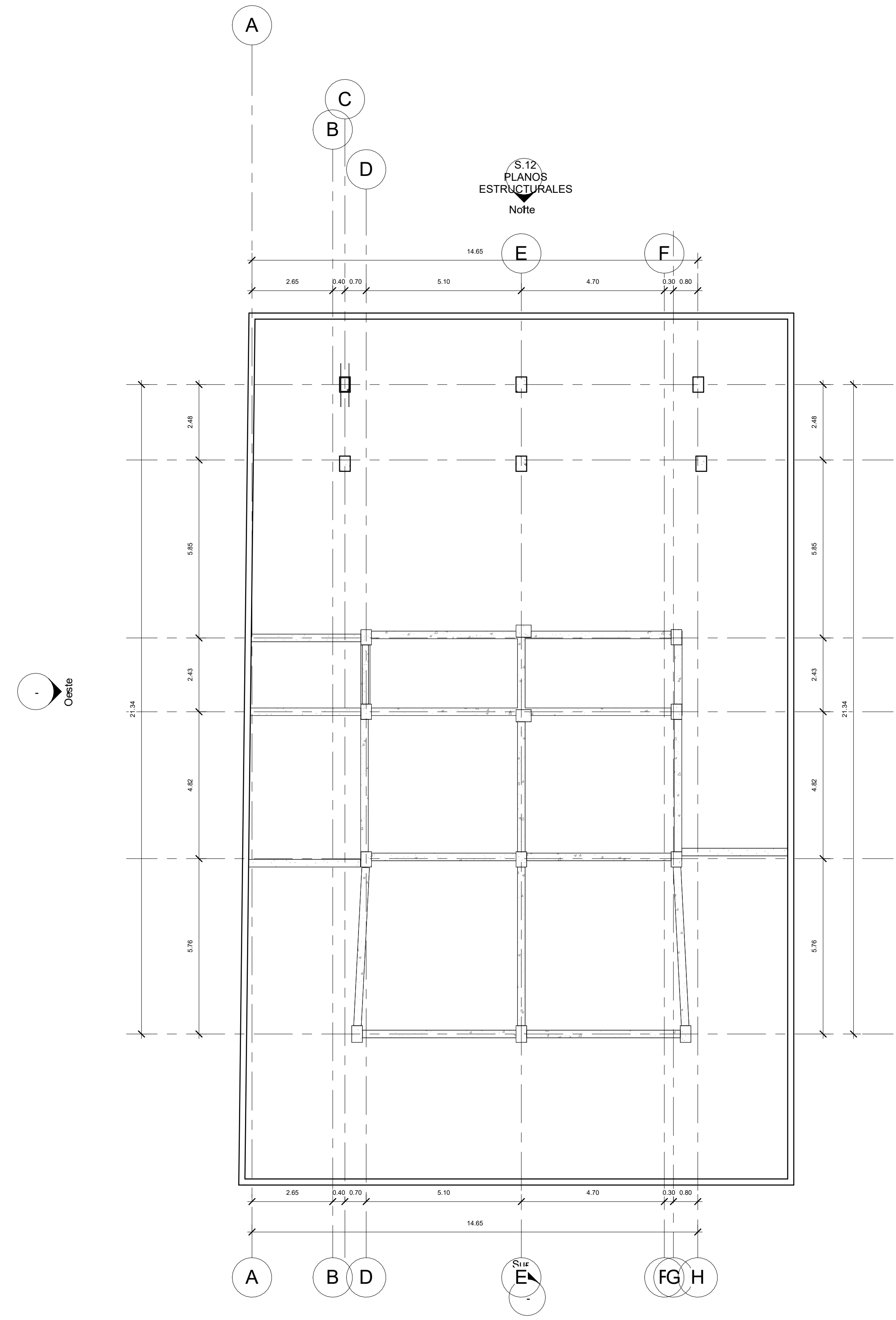
1 N-3.12 Subsuelo 1 1 : 100
