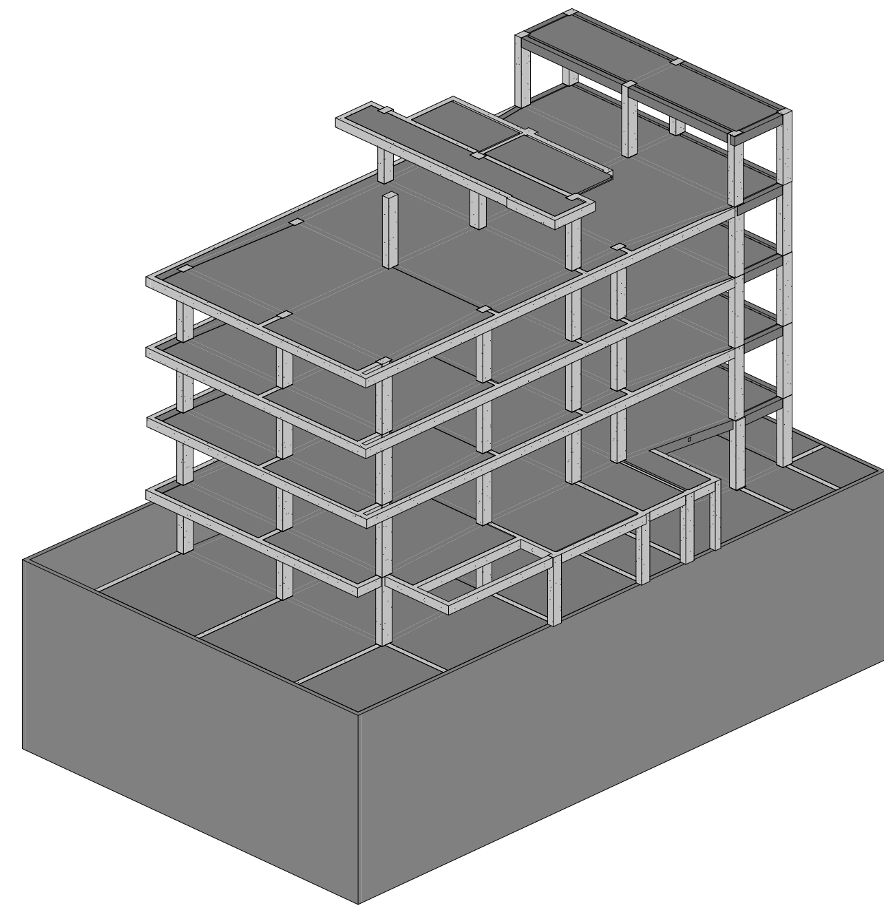
2 Modelo analítico
