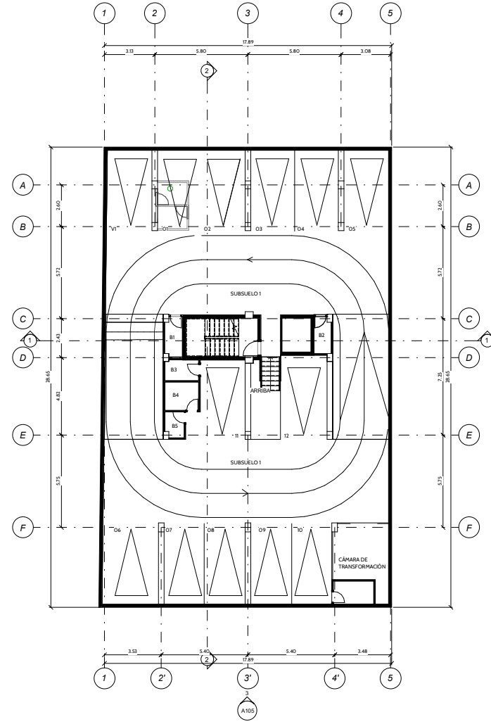
2 - 024-Subsuelo 1 A3(1) 1:100
