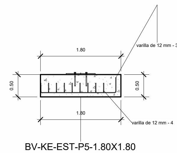
4 Sección 1 CIMENTACION 1 : 50
