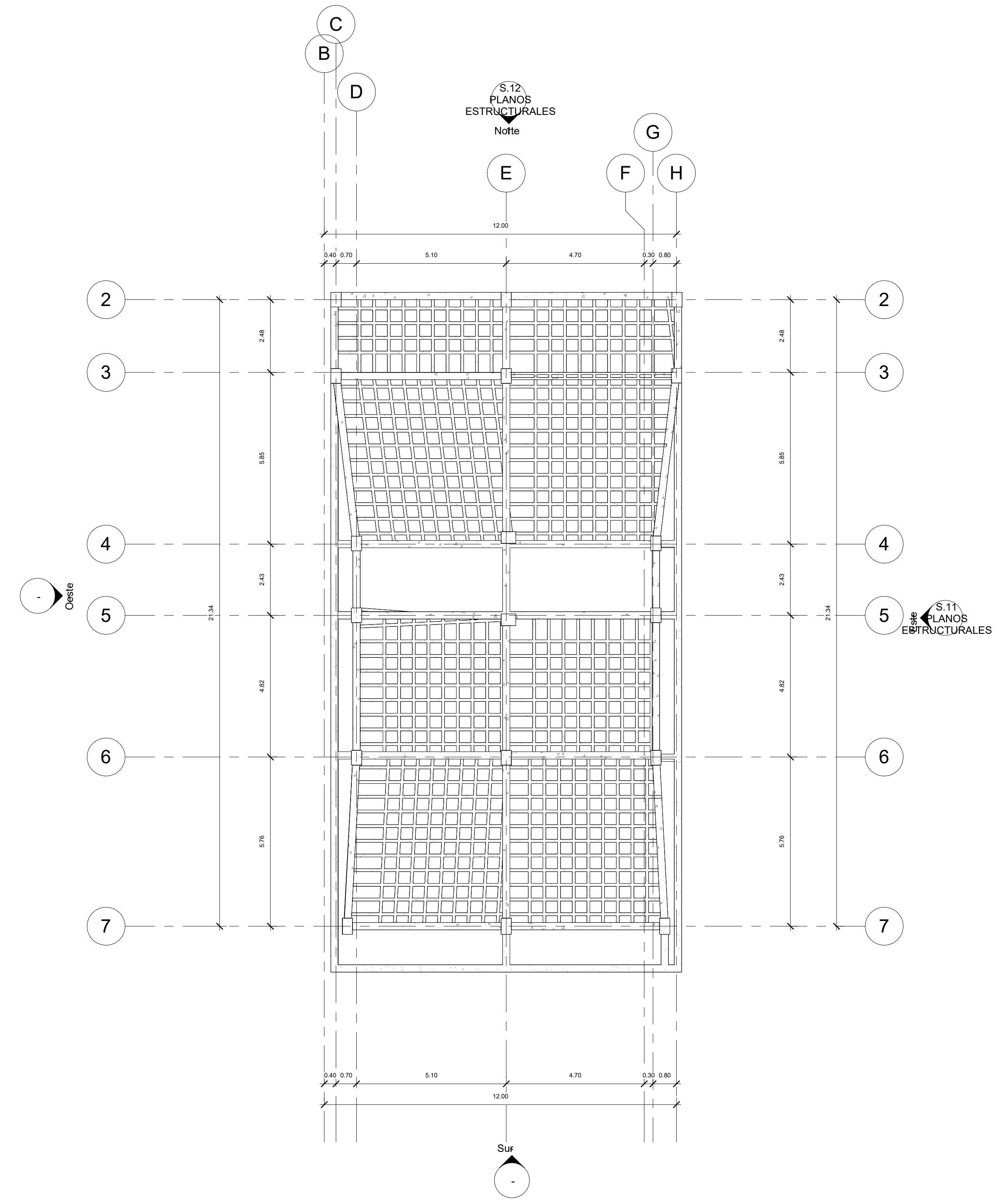
1 Nivel 4 1 : 100
