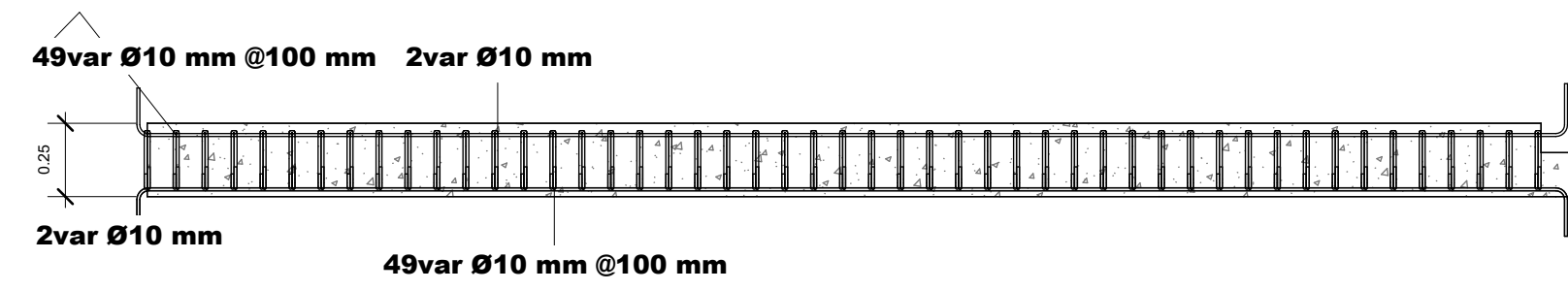
2 Nivel 1 -DETALLE DE VIGA 1 : 25
