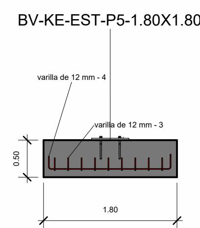
6 DETALLE DE PLINTO 1 : 50
