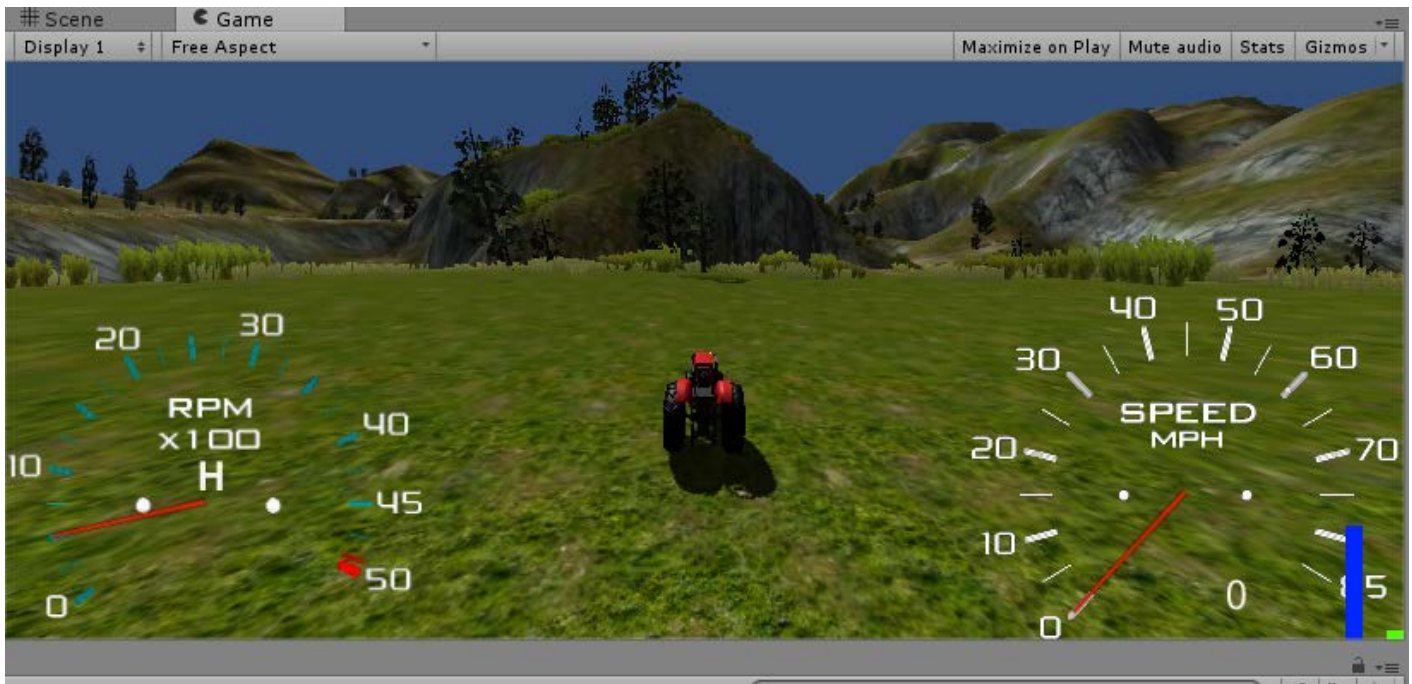
Imagen 6. Escena virtual.
