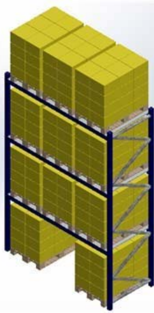
2. Ensamblaje de la estantería simple
