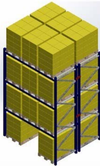
3. Ensamblaje de la estantería doble
