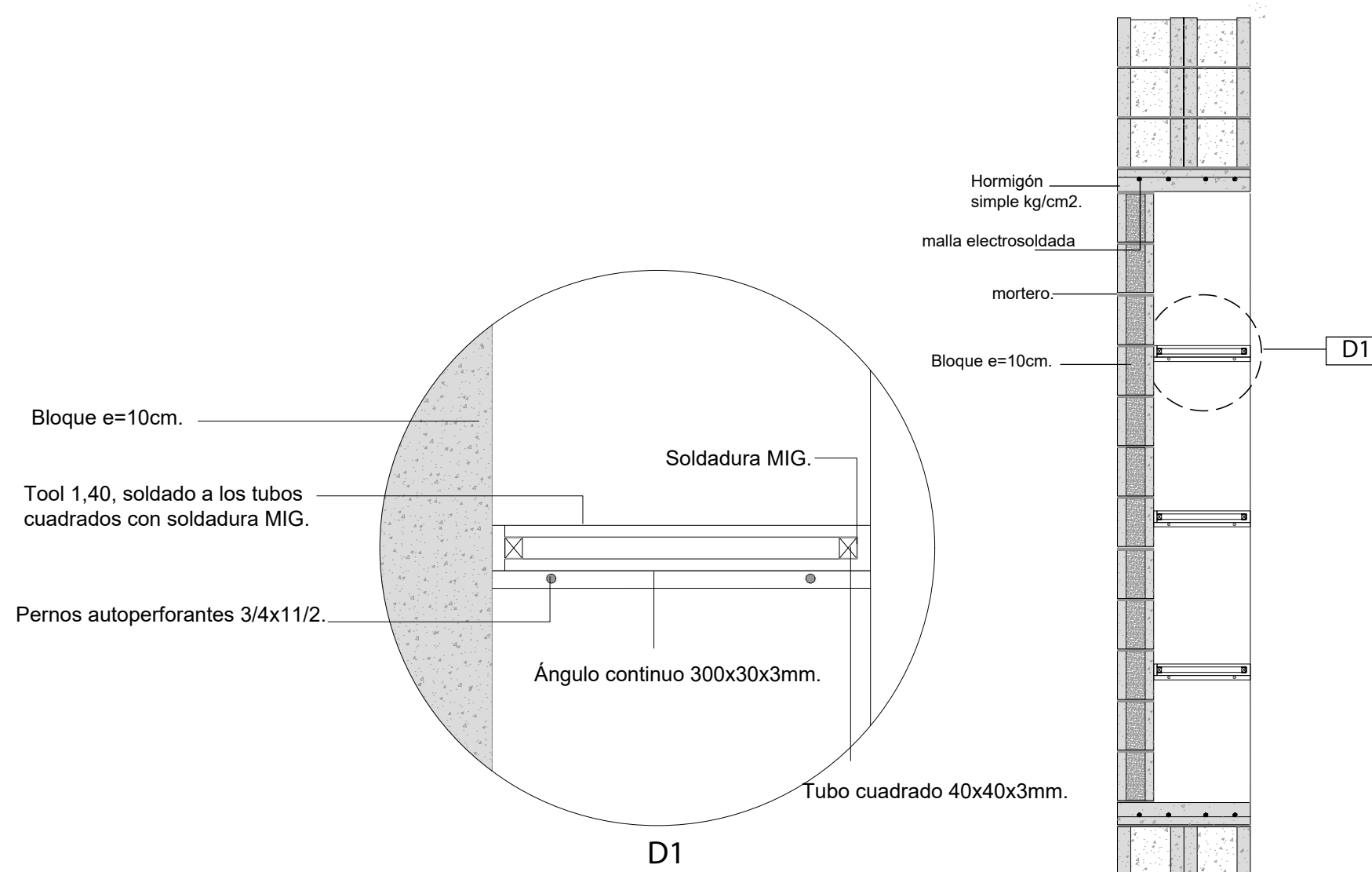
Detalle Constructivo 2 Librero Escala 1:25
