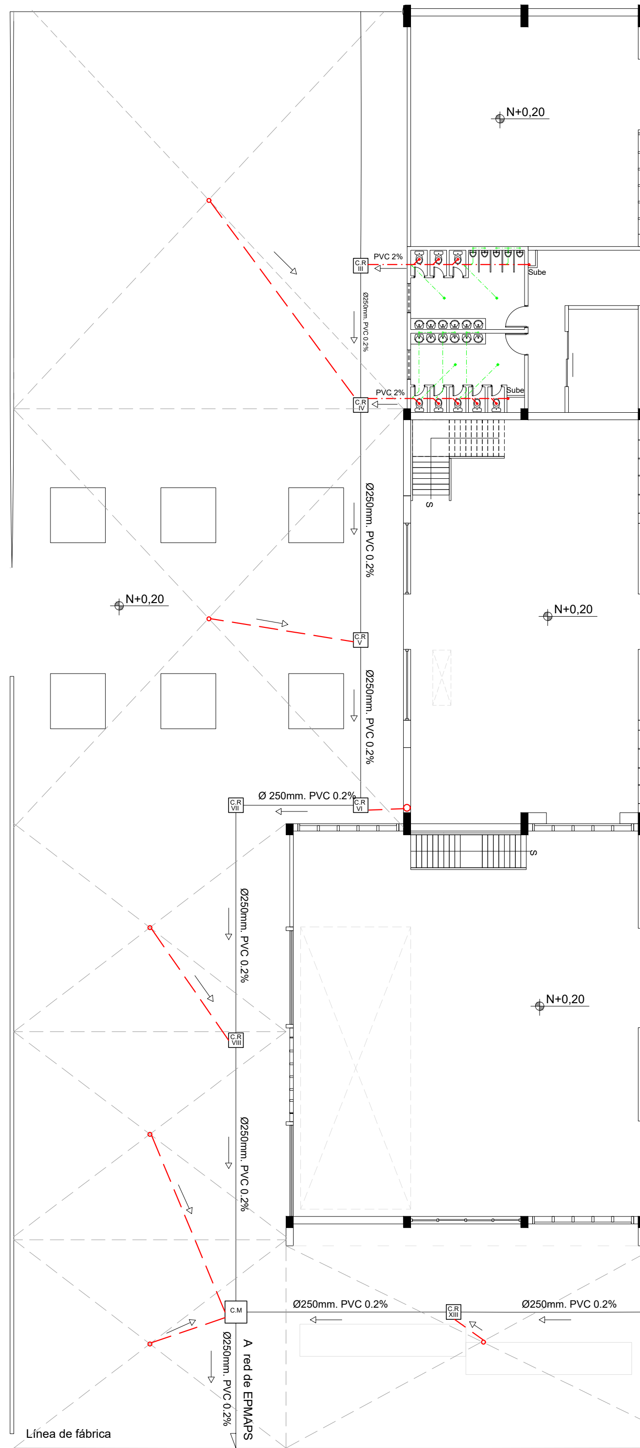
Instalaciones Hdrosanitarias Aguas servidas Escala 1:200
