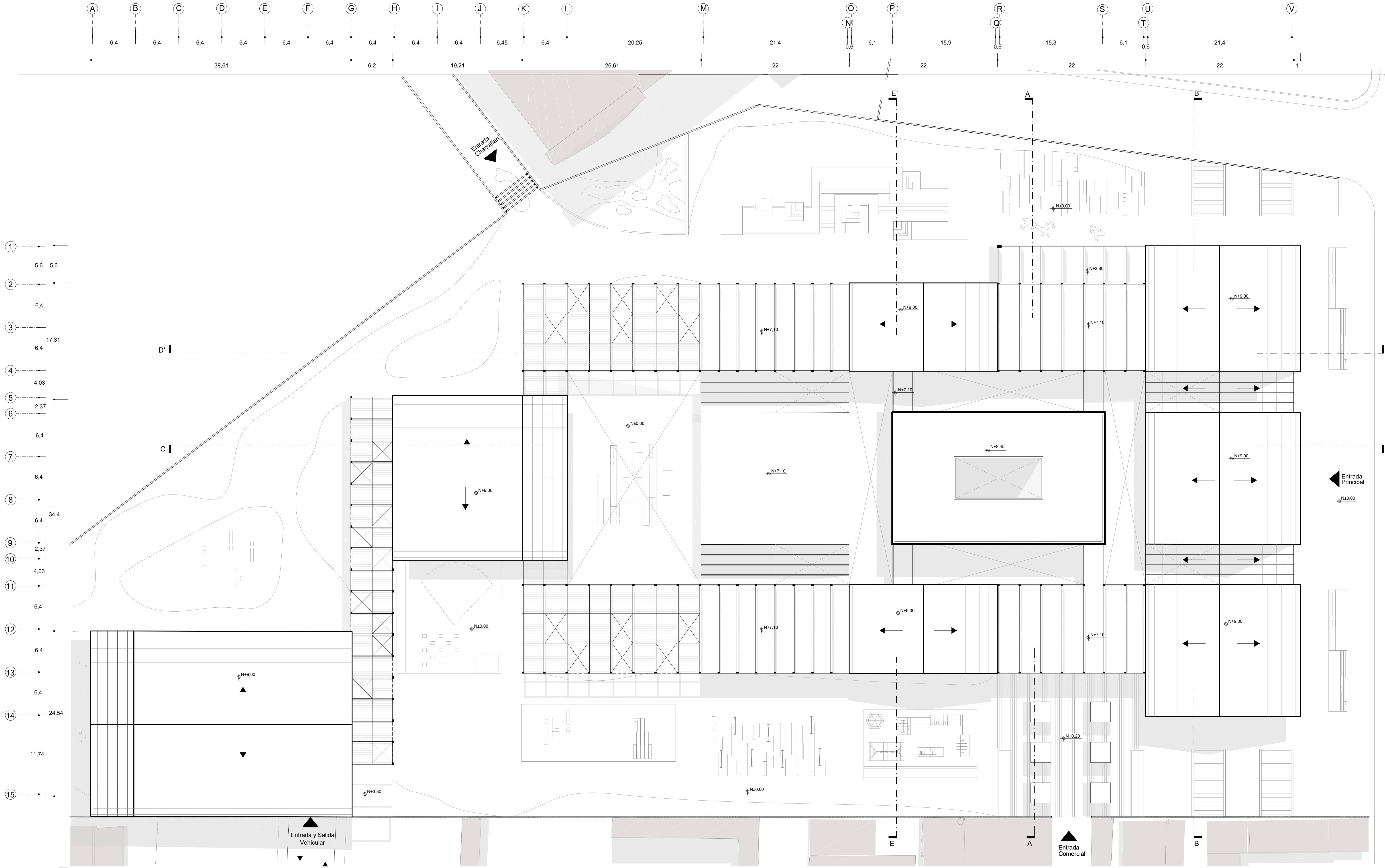
Planta de cubiertas Escala 1:250
