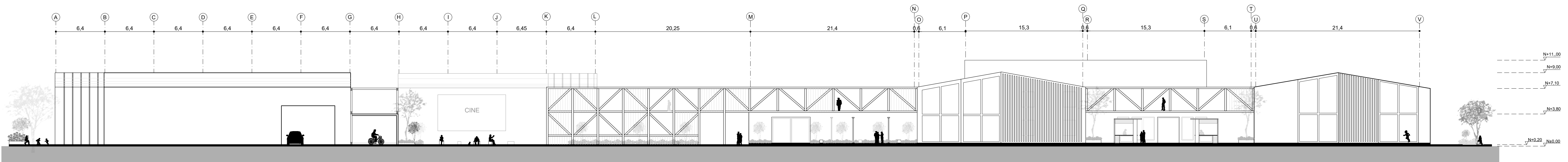
LT. 4. Elevación Suroeste Escala 1:250
