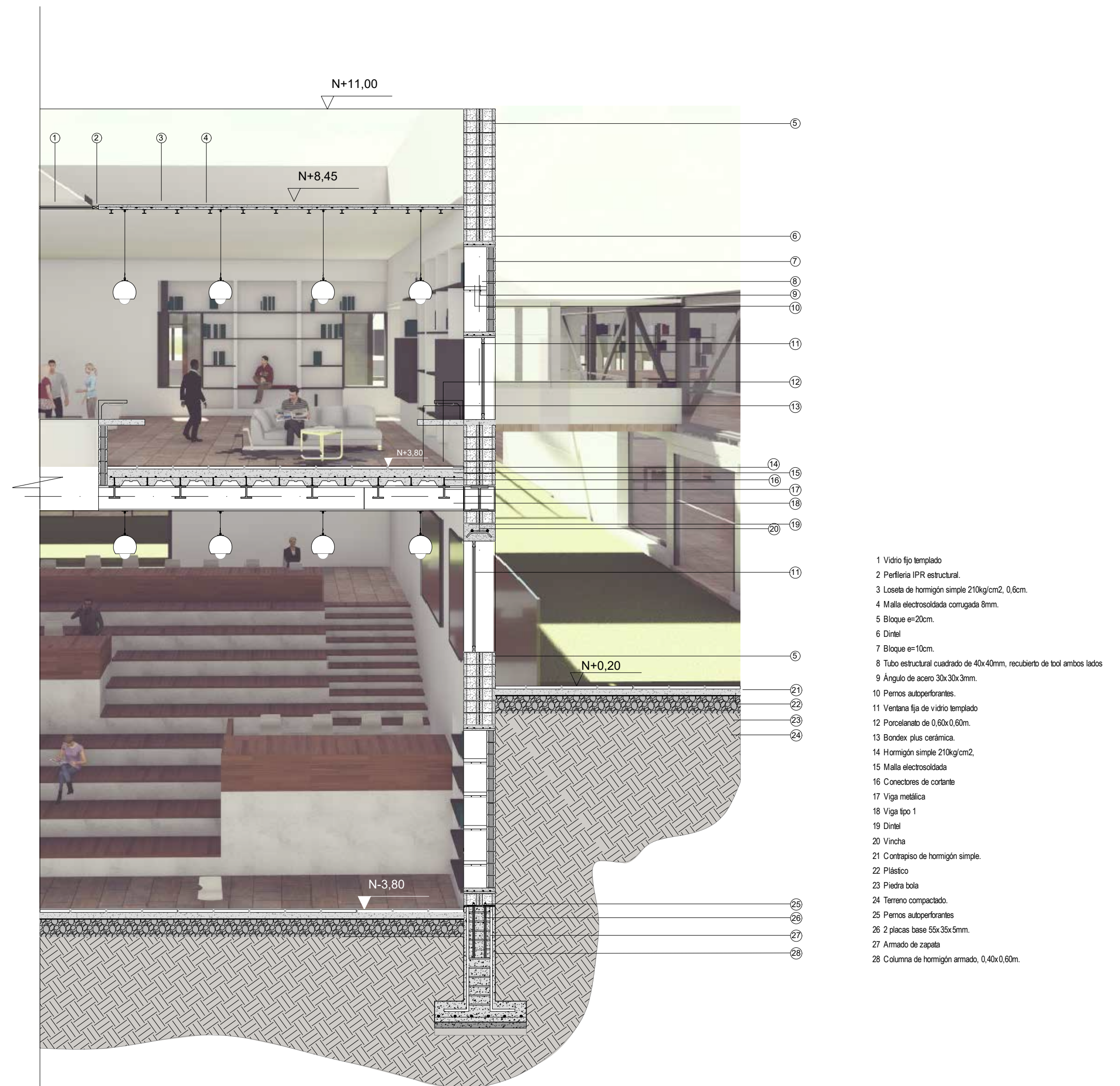
Detalle Arquitectónico 3 Escala 1:75
