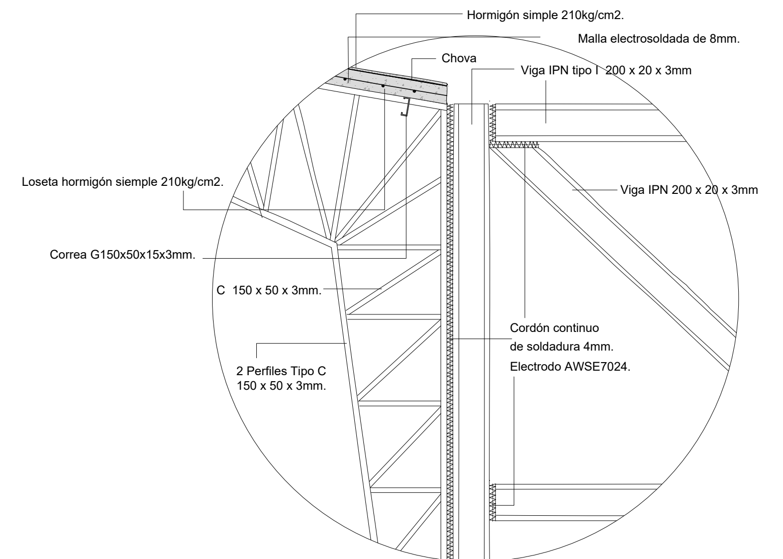
Detalle Constructivo 4 Unión de columnas con vigas puente Escala 1:25
