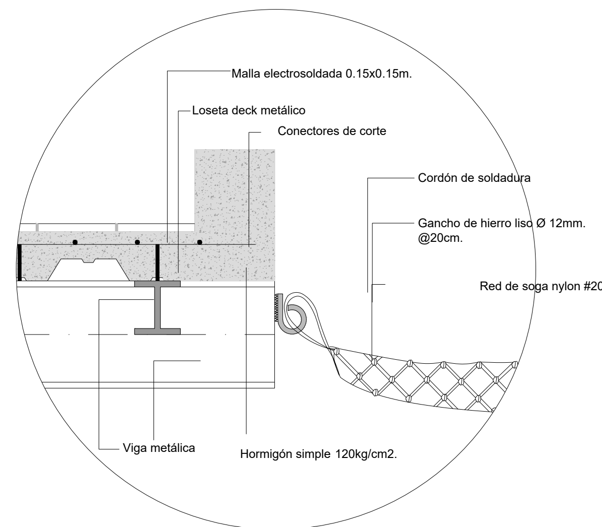
Detalle Constructivo 3 Red Escala 1:25
