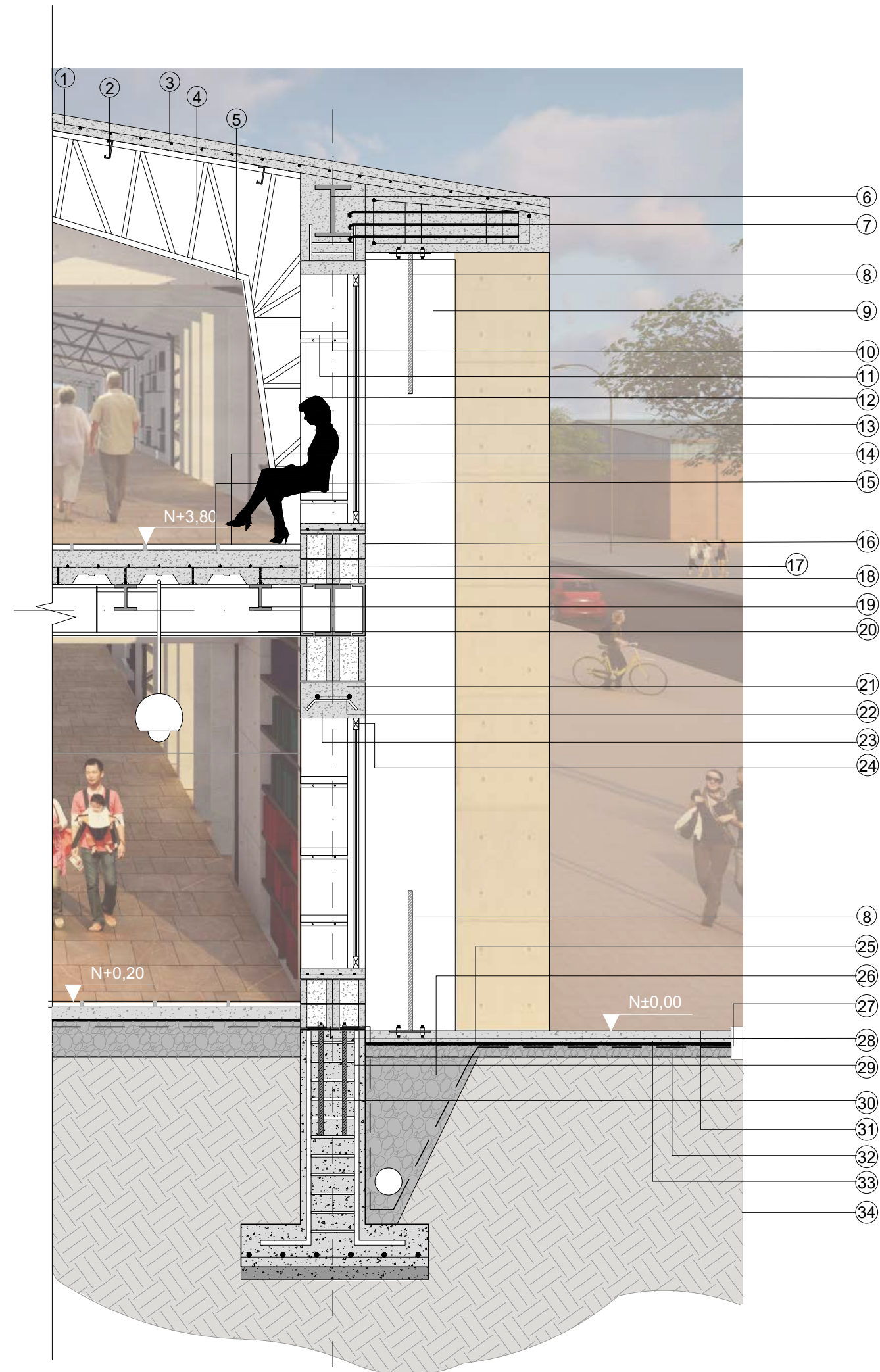
Detalle Arquitectónico 1 Escala 1:50
