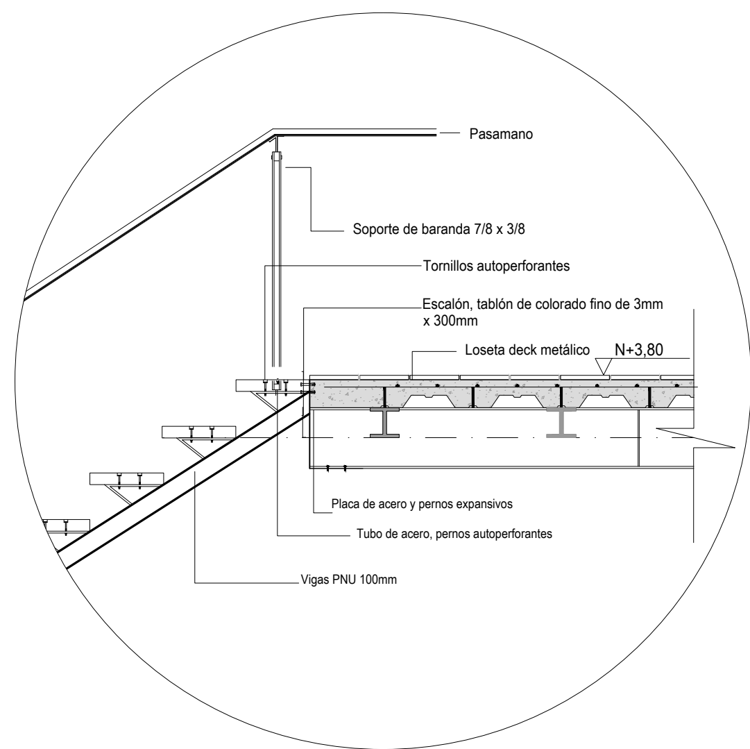
Detalle Constructivo 1 Escalera Escala 1:25
