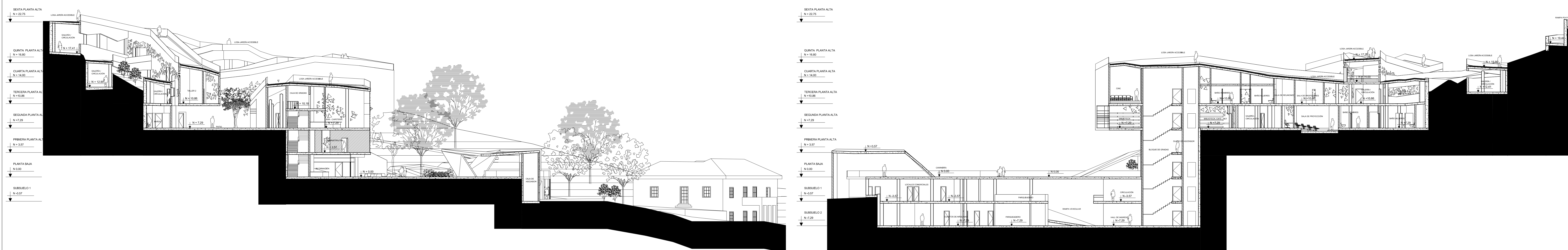
CORTE E-E'
