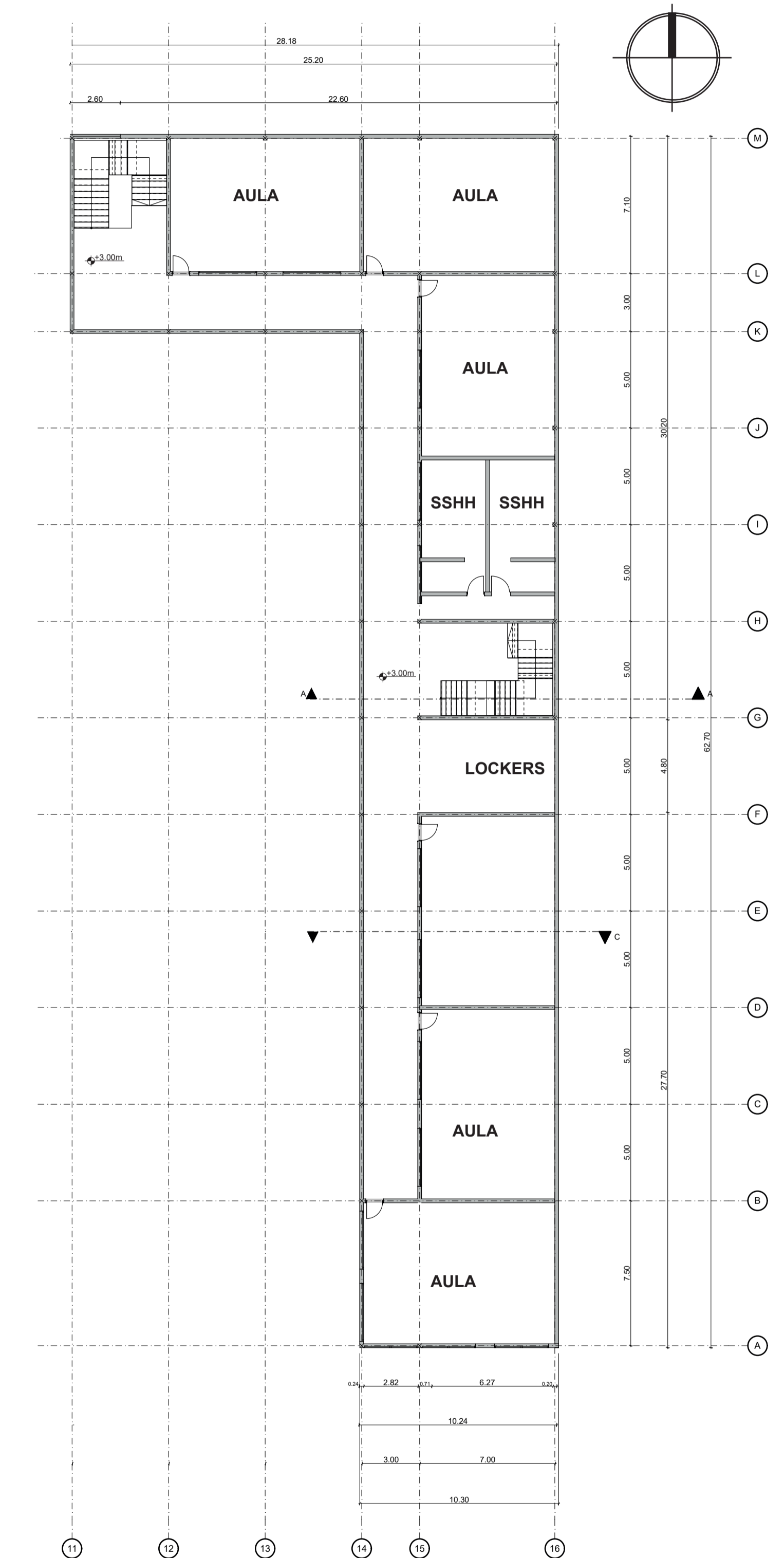
0. PLANTA ALTA 1:200
