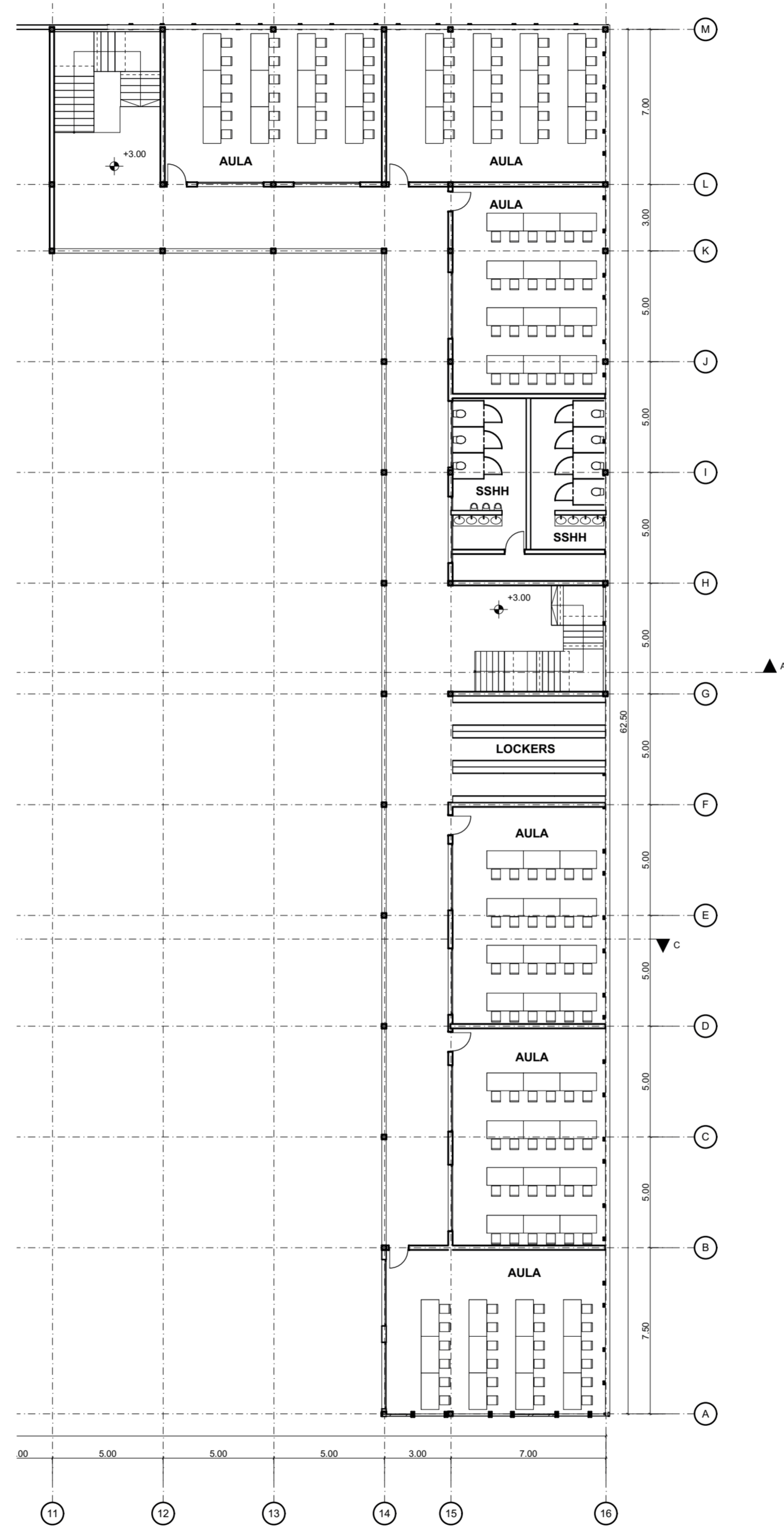
1. Planta Alta 1:200
