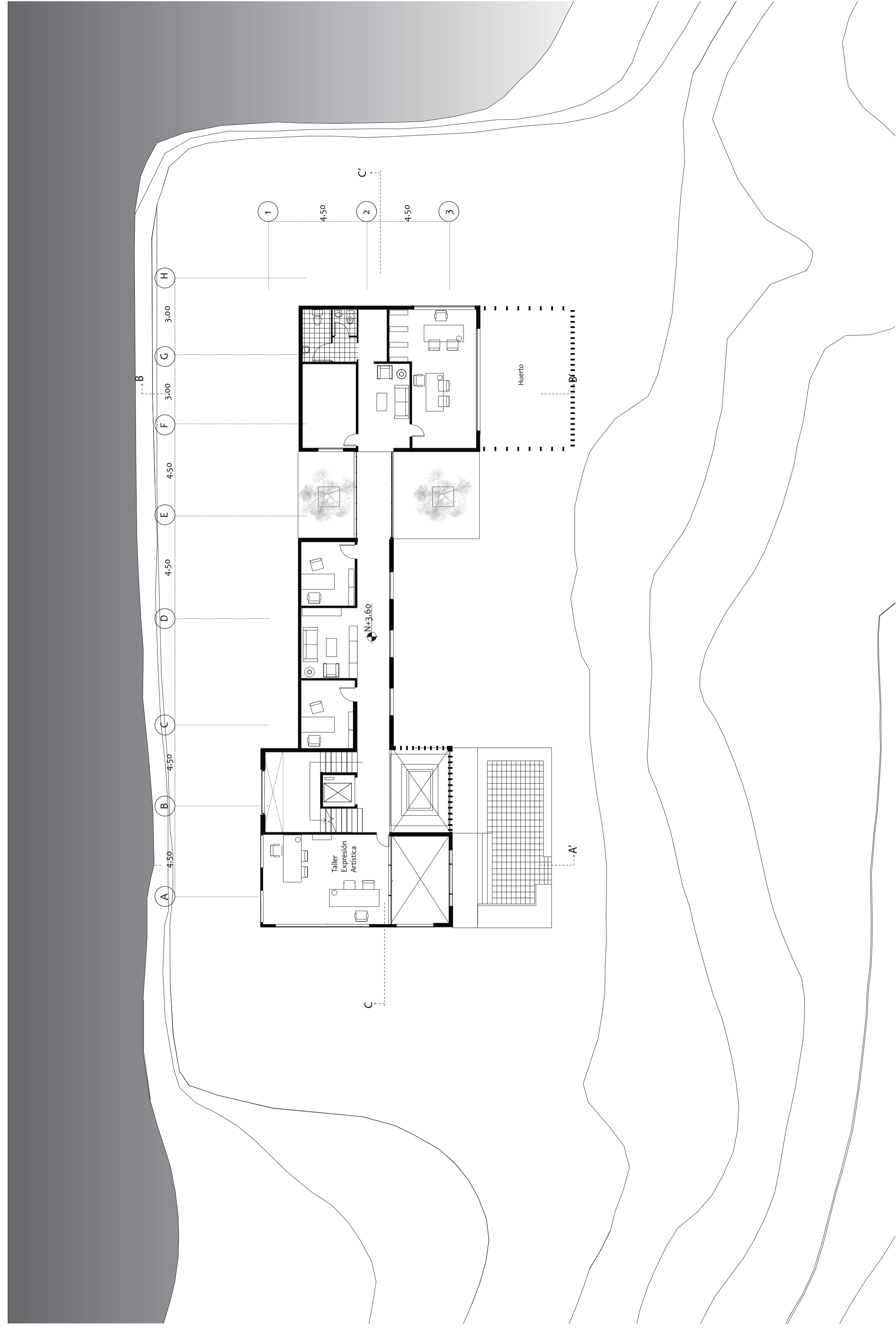
Planta Nivel +3.06
