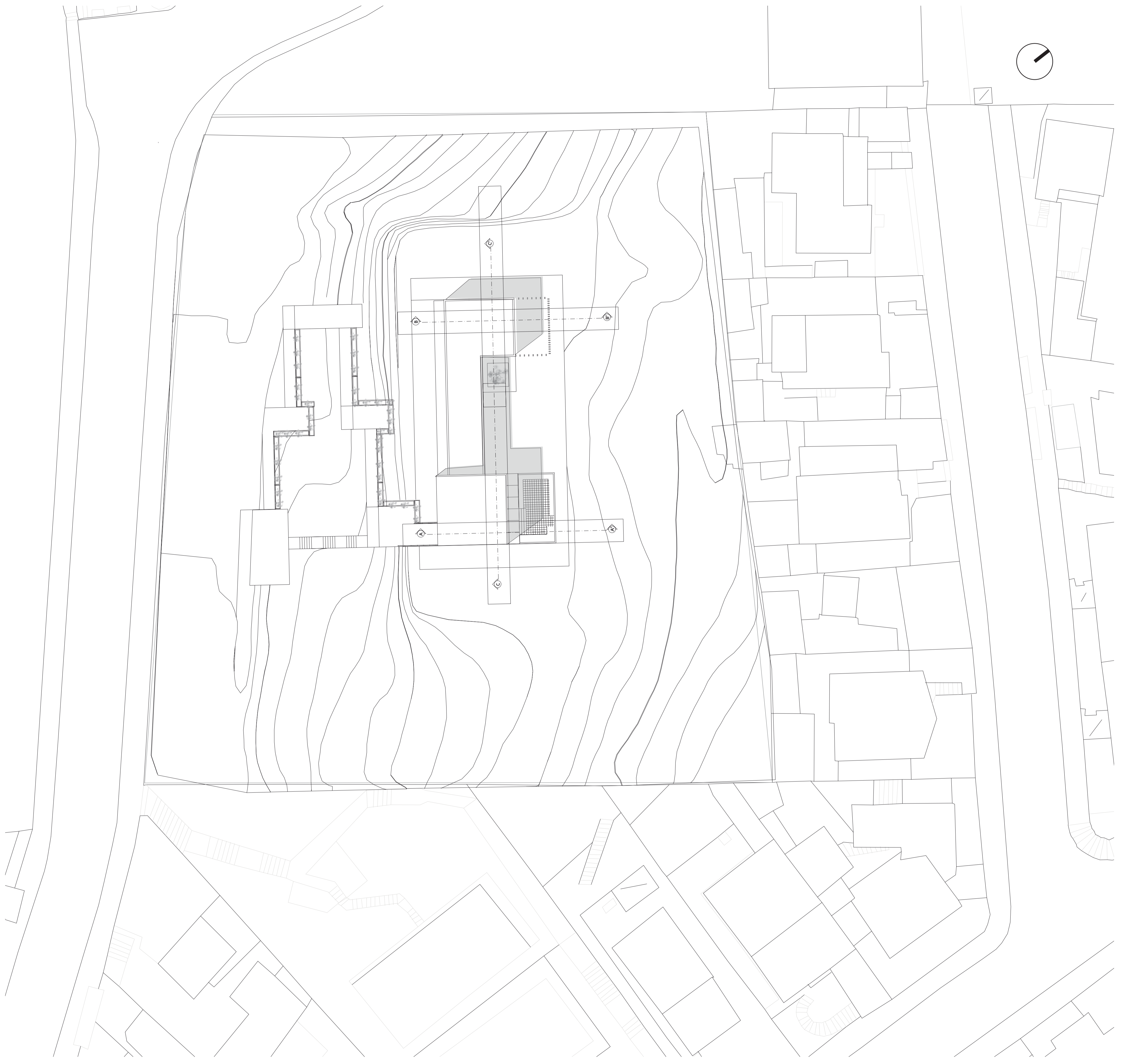
Implantación General
