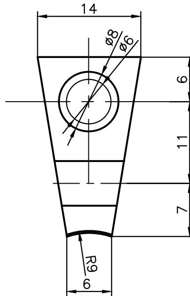
VISTA FRONTAL ESC 2:1
