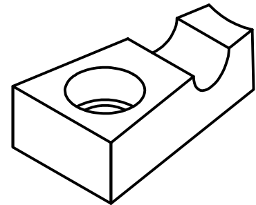
VISTA ISOMETRICA ESC 2:1
