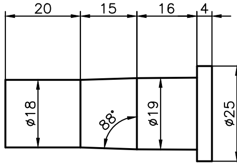
VISTA LATERAL ESC 1:1
