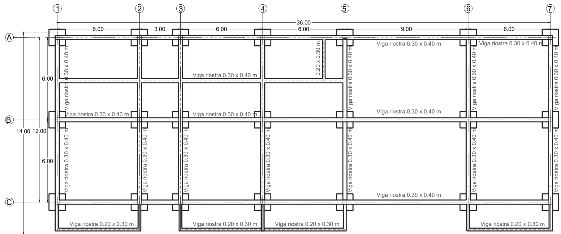
Planta de Esquema Estructural
