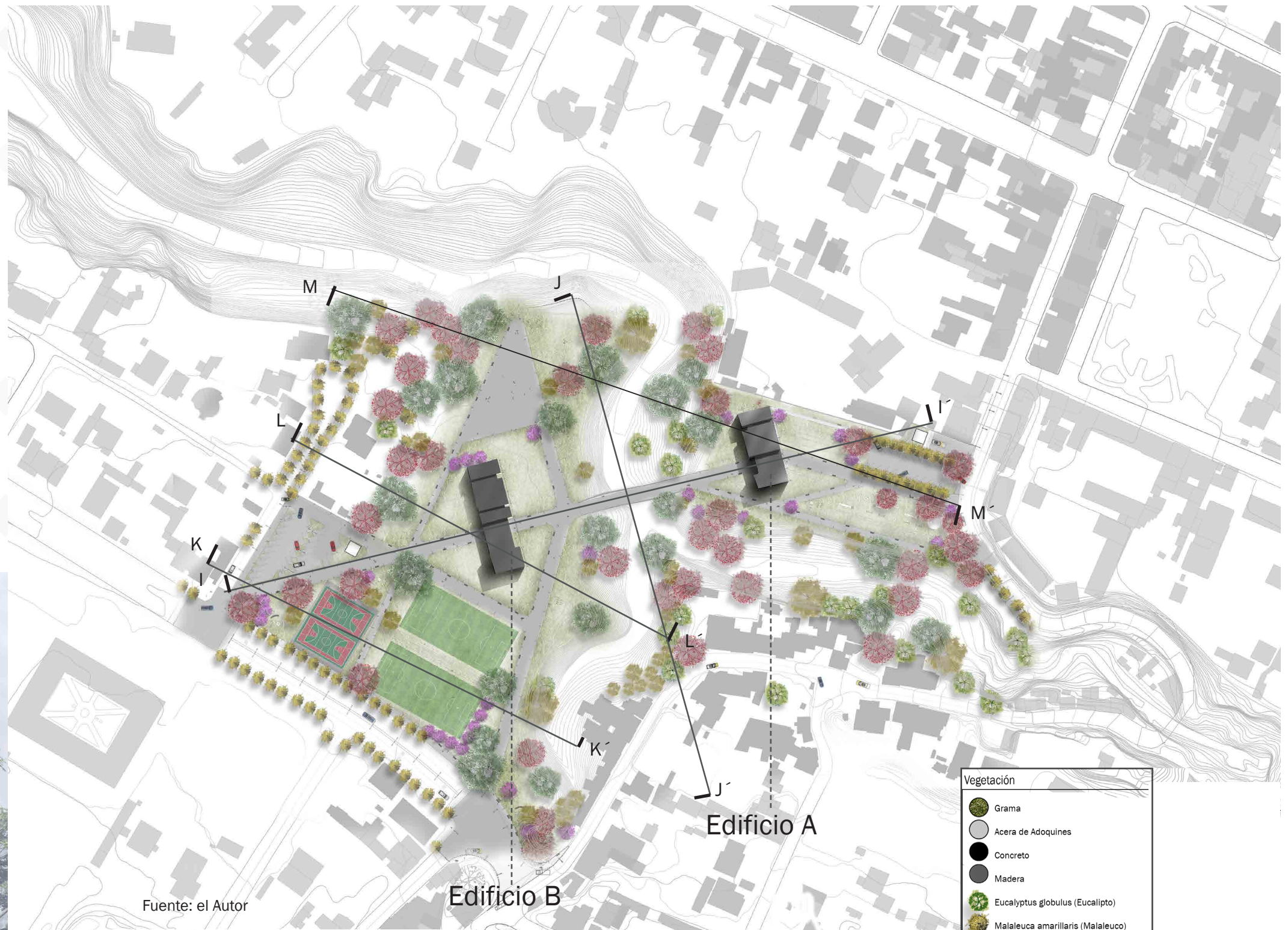
Planta General del Conjunto
