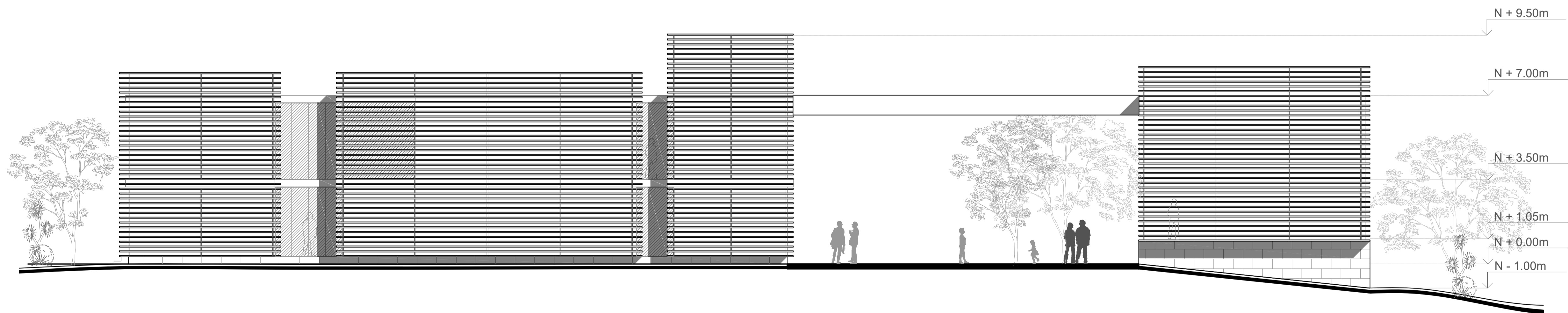
Fachadas Noreste
