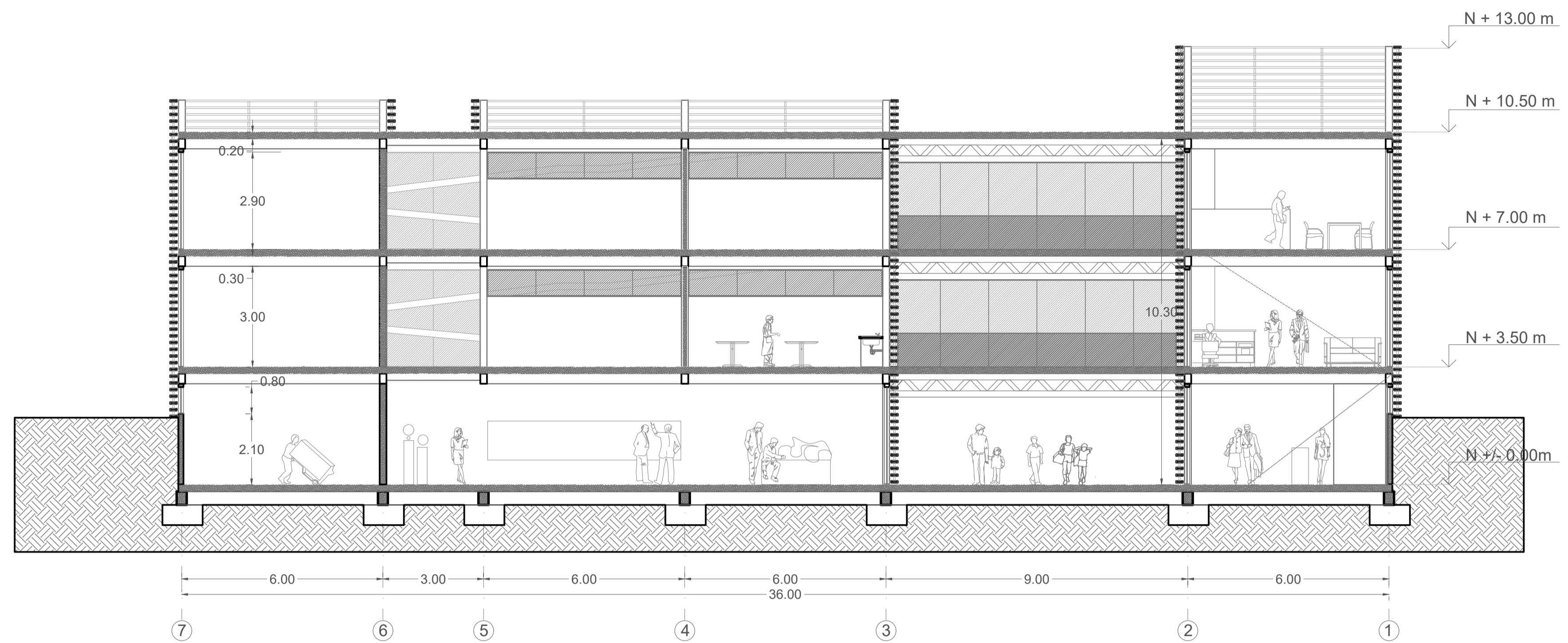
Corte C-C'
