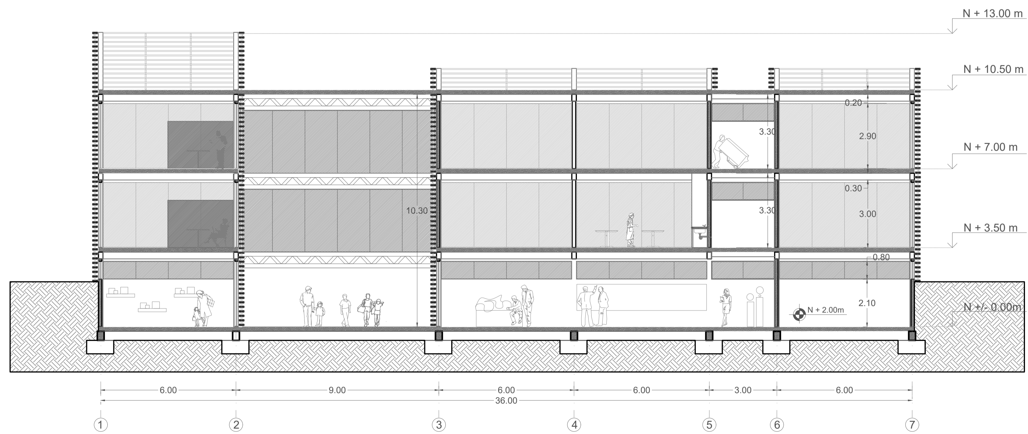
Corte D-D'
