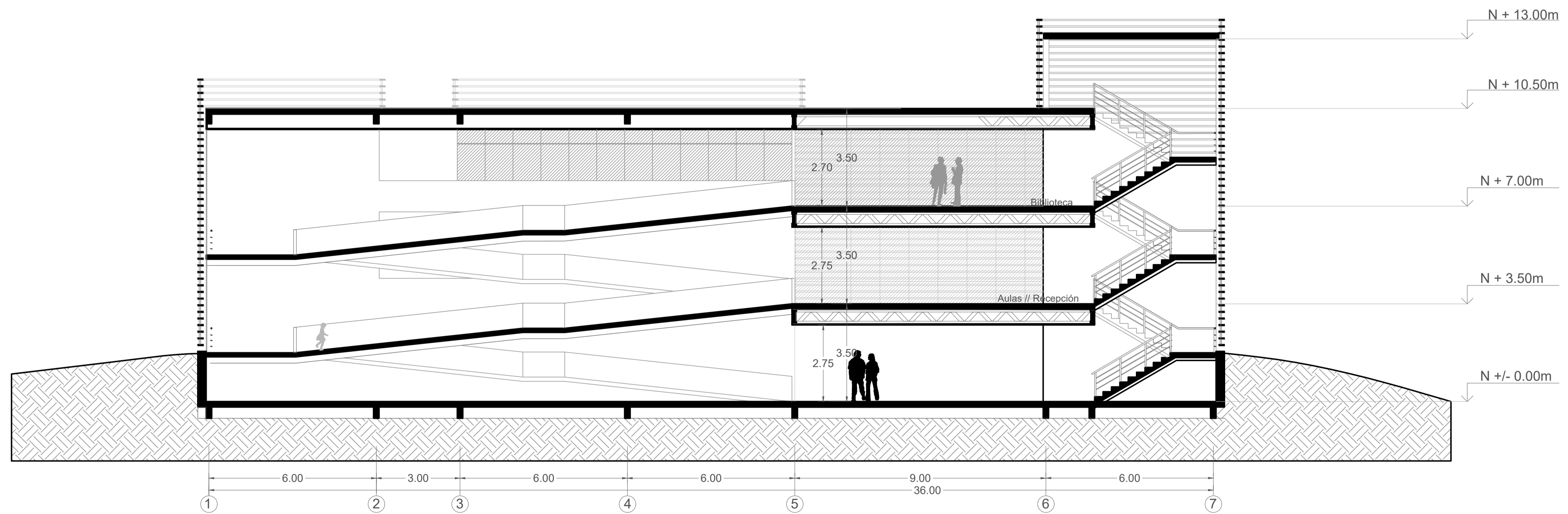
Corte B-B'
