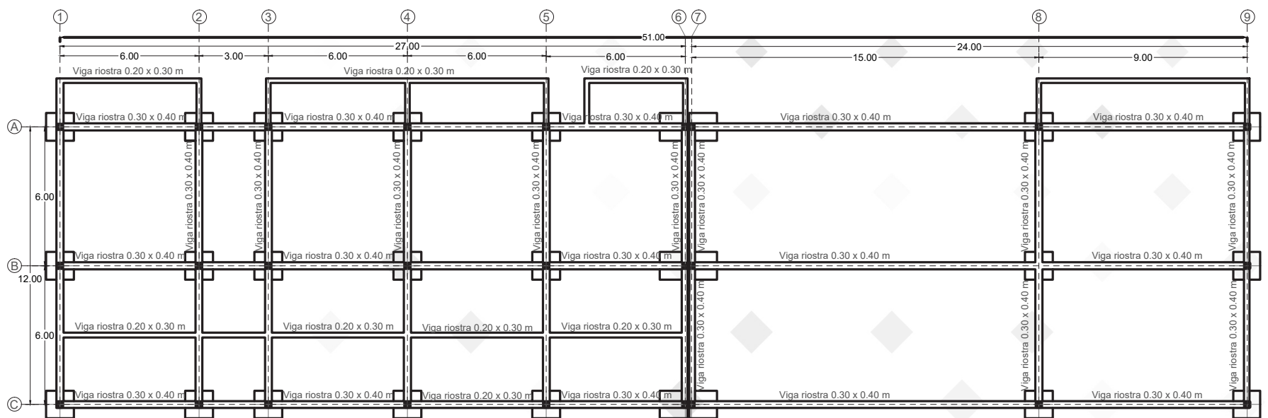
Planta Estructural
