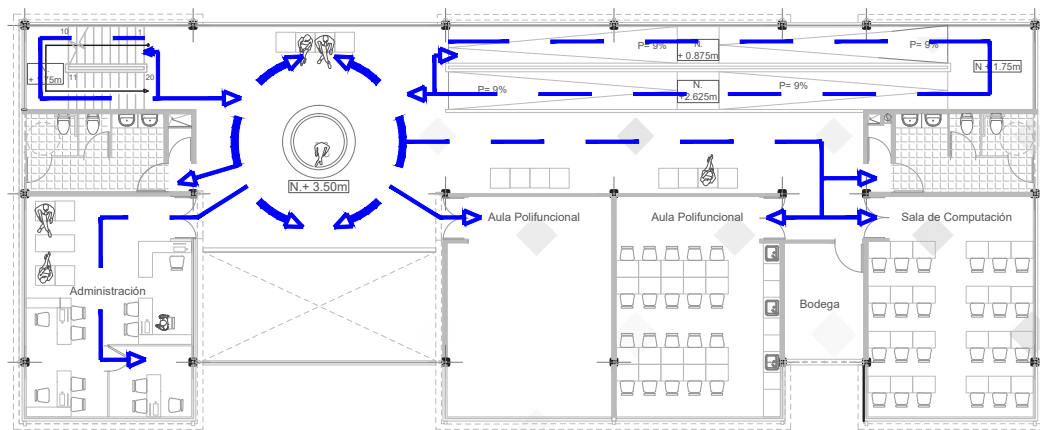
PLANTA NIVEL N. +7.50 m
