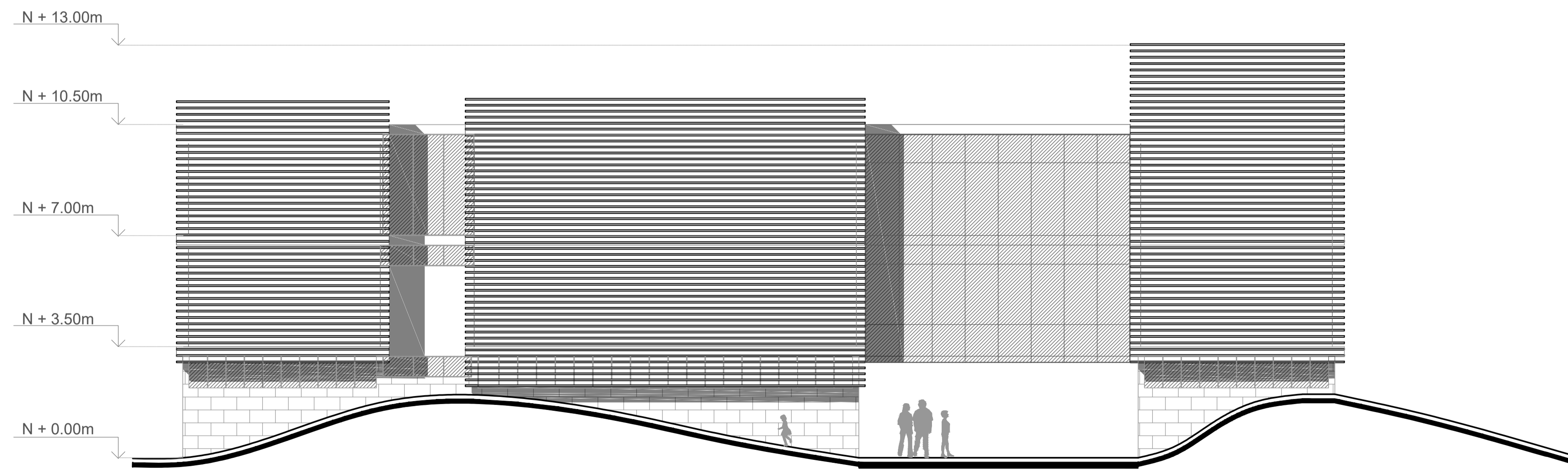
Fachadas Suroeste
