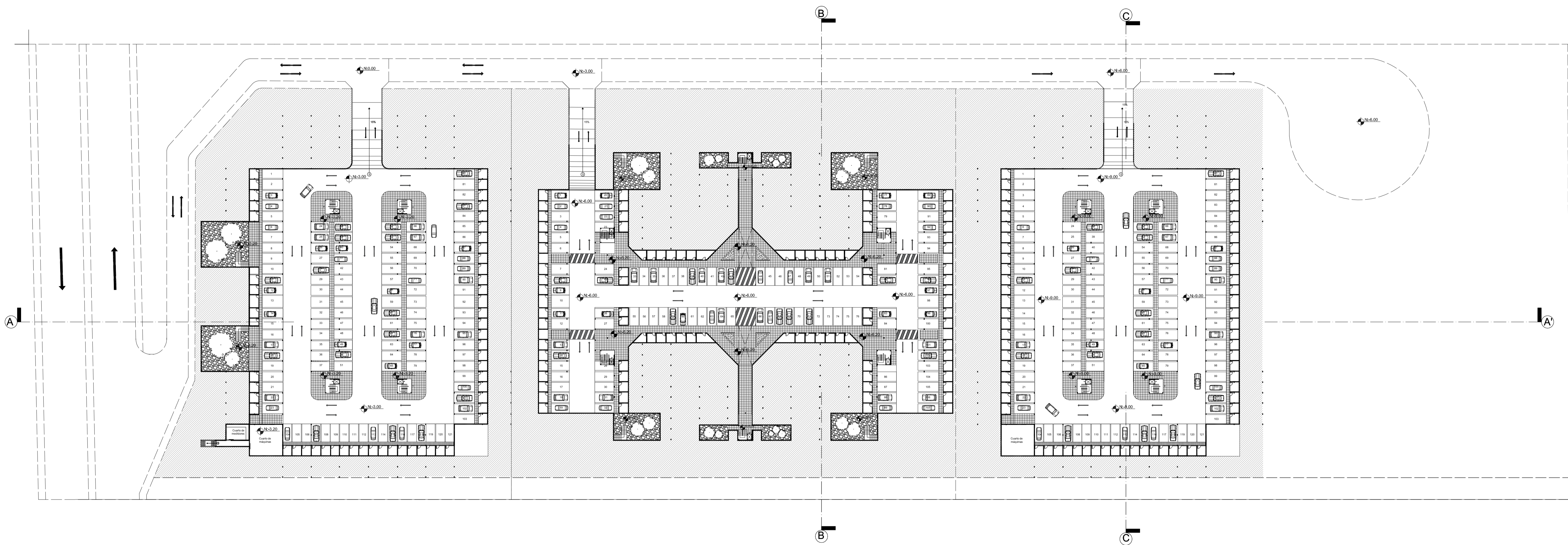
PLANTA DE SUB SUELO E_ 1:500
